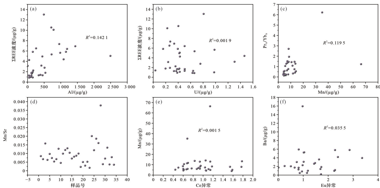
图4 元坝地区早三叠世飞仙关组二段鲕粒和巨鲕陆源碎屑和成岩作用影响评价
