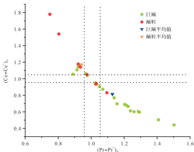
图9 元坝地区早三叠世飞仙关组二段鲕粒和巨鲕 (Pr/Pr^*)_N 和 (Ce/Ce^*)_N 交会图
