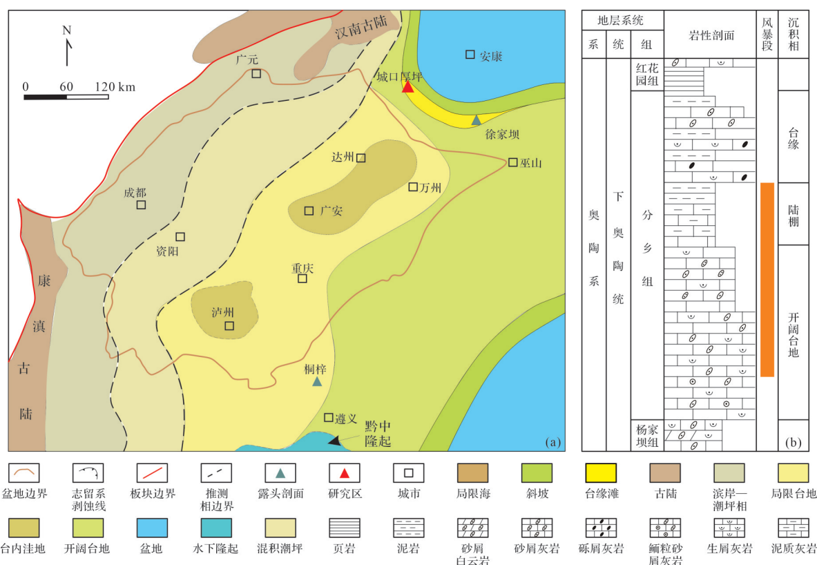
图1 (a)四川盆地早奥陶世岩相古地理;(b)厚坪剖面分乡组地层柱状图(据文献[35]修改)
