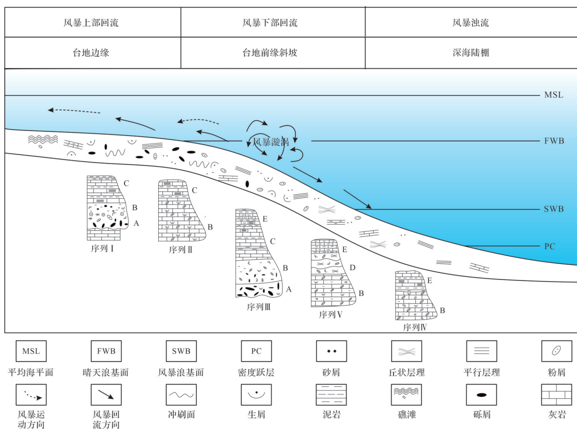
图5 城口地区下奥陶统分乡组风暴沉积模式图
