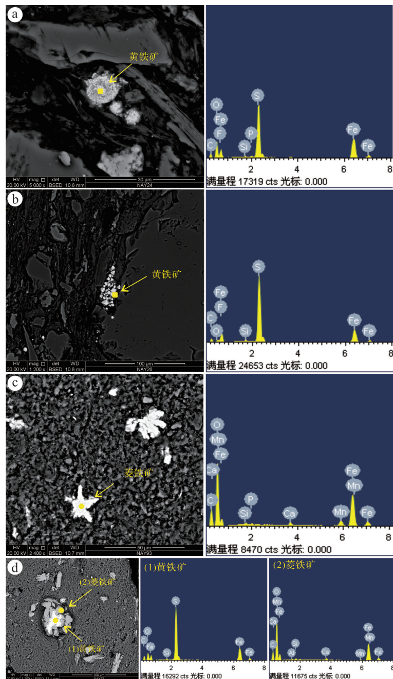
图4 安崖样品扫描电镜图像
