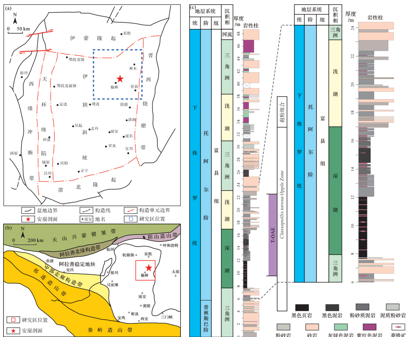
图1 鄂尔多斯盆地构造及研究区位置剖面 and 岩性划分
