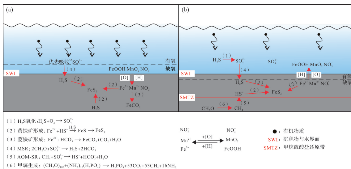
图8 安崖剖面 Toarcian 期硫同位素控制模型
