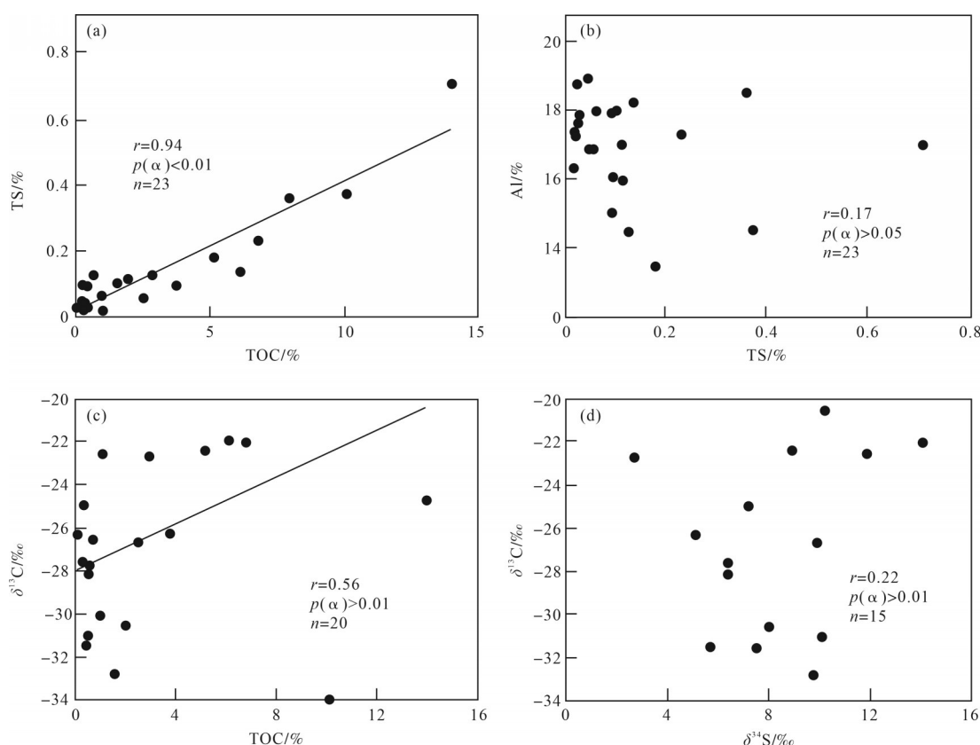
图5 安崖样品各地球化学参数相关性图
