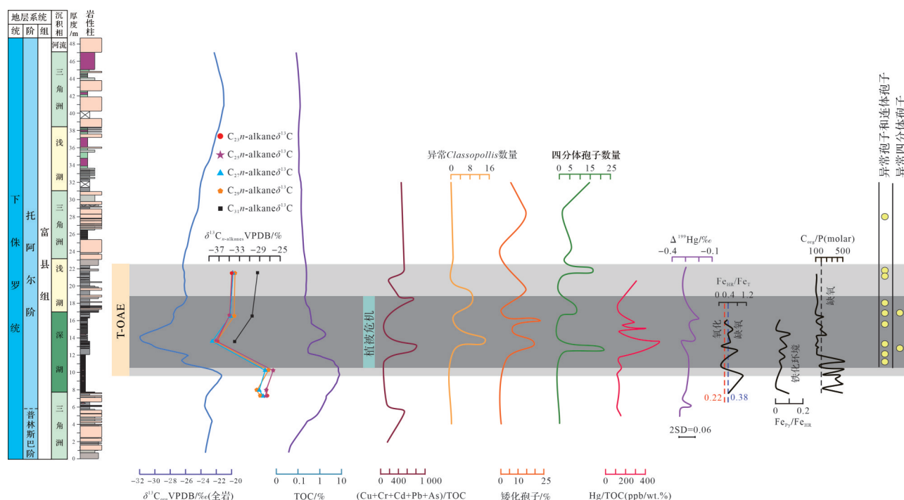
图2 安崖剖面T-OAE时期生物—环境变化
