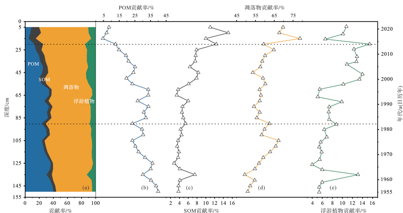
图7 柱状沉积物中有机碳潜在来源贡献率及其分布特征
