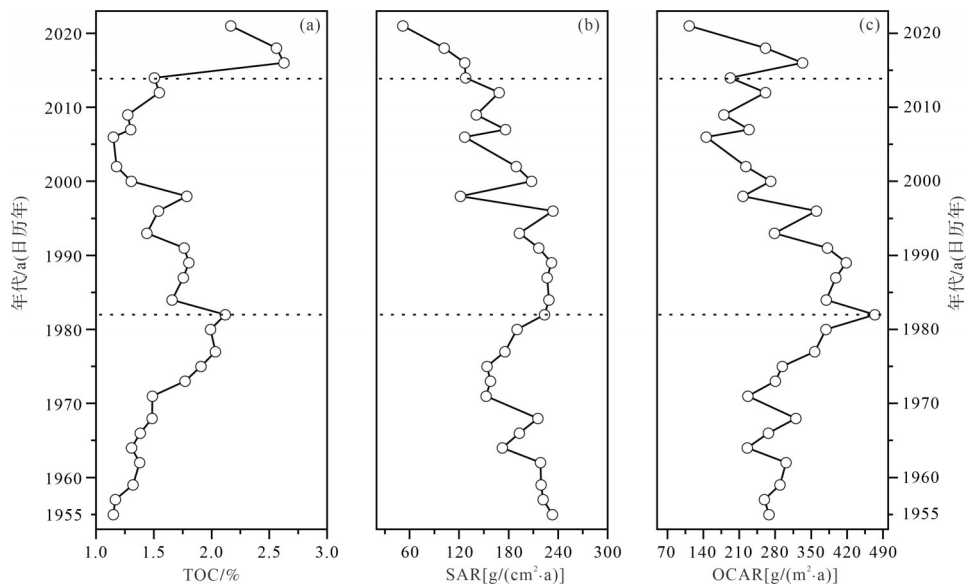
图4 柱状沉积物中 TOC、SAR、OCAR 的垂直分布
