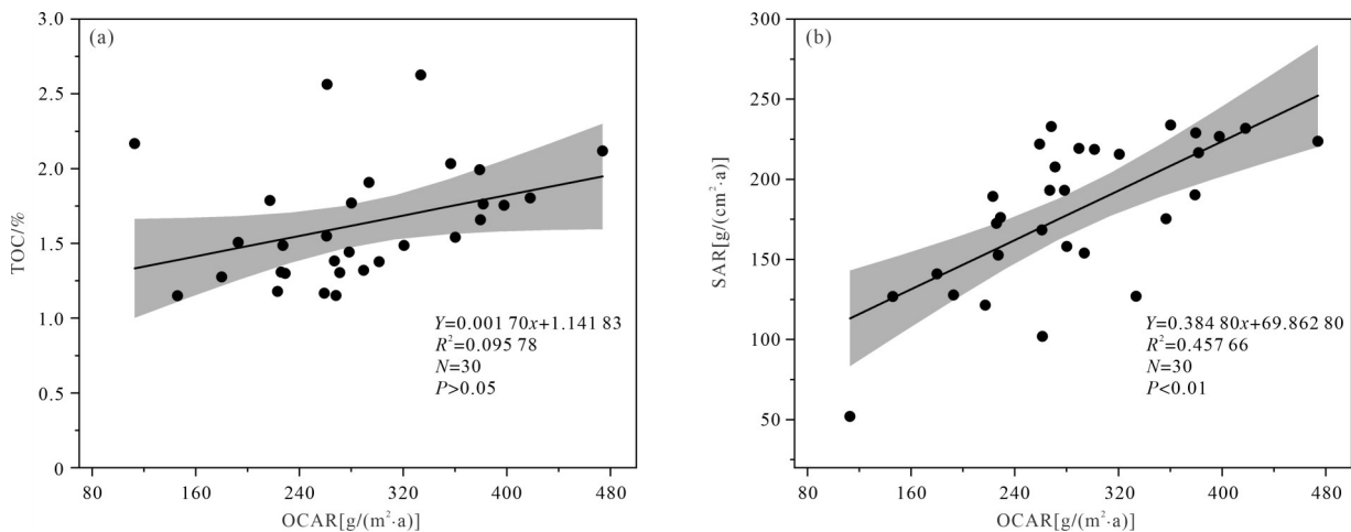
图5 柱状沉积物中 OCAR 与 TOC/SAR 的相关关系
