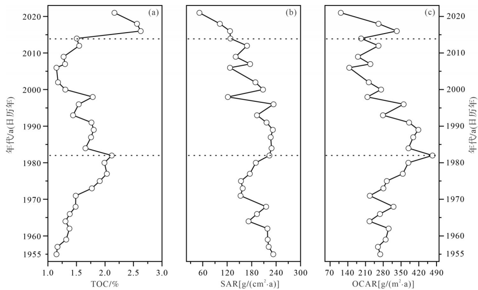
图4 柱状沉积物中 TOC、SAR、OCAR 的垂直分布
