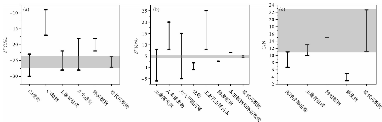
图6 柱状沉积物中 \delta^{13}\text{C} 、 \delta^{15}\text{N} 和C/N的来源分布特征
