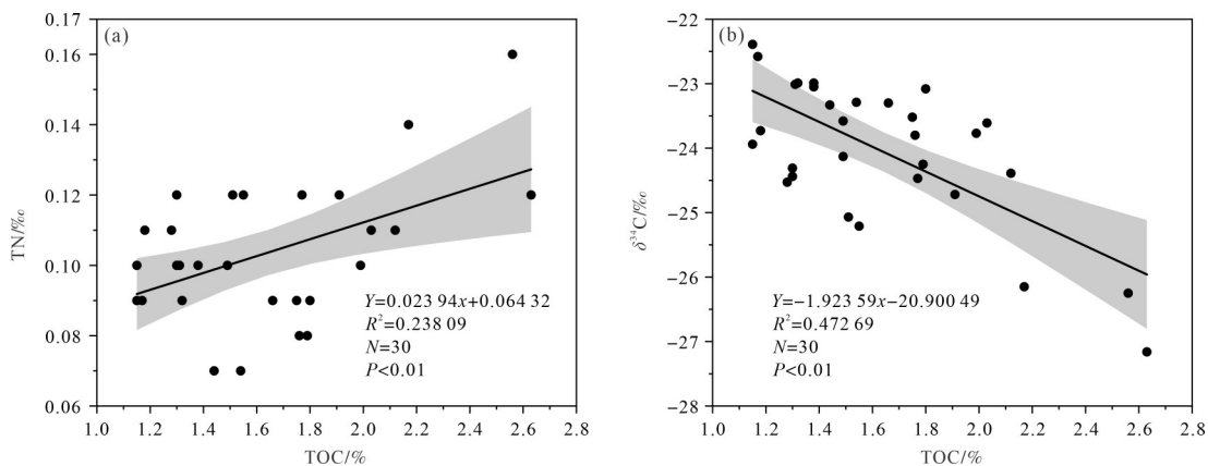
图3 柱状沉积物中TOC与TN/ \delta^{13}\text{C} 的相关关系
