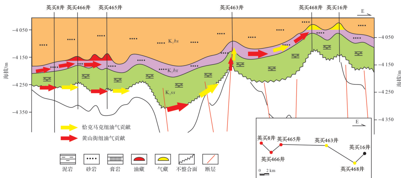
图 14 油气运移模式图(据文献[29]修改)
