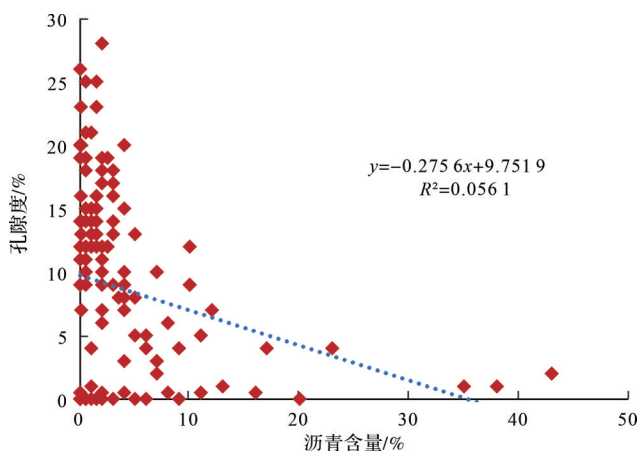
图 15 储层沥青含量与孔隙度拟合关系曲线
