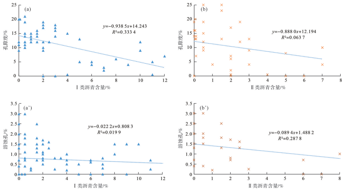
图 16 不同沥青类型与孔隙类型的关系散点图 (a,a') I类沥青含量与孔隙度、溶蚀孔关系;(b,b') II类沥青含量与孔隙度、溶蚀孔关系
