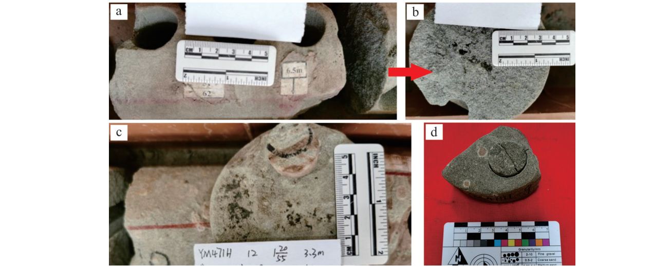
图4 塔北西部白垩系巴西改组中沥青岩心观察特征 (a)英买467井,5 200.40 m,巴西改组,见少量斑状沥青;(b)英买467井,5 200.40 m,巴西改组,见少量斑状沥青(视图放大);(c)英买471H井,5 202.35 m,巴西改组,见点状沥青分布;(d)英买471H井,5 197.50 m,巴西改组,沥青呈黑色小点均匀分布于颗粒间 Fig.4 Observation characteristics of bitumen cores from the Cretaceous Baxigai Formation in the western Tabei area
