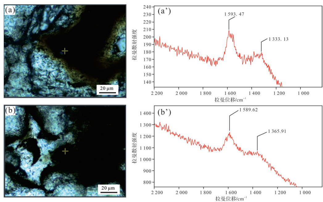
图6 不同类型沥青激光拉曼光谱特征
