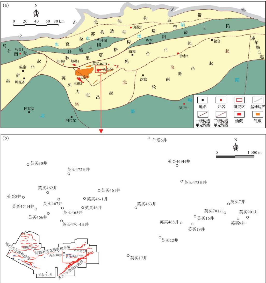
图1 研究区区域概况图(据文献[24]修改)
