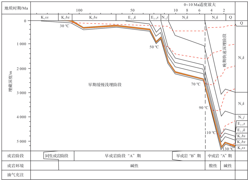
图 17 巴西改组成岩演化序列(据文献[48]修改)
