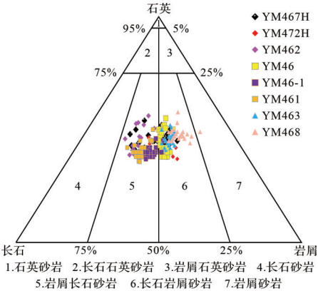
图3 英买467井区巴西改组岩性三角图
