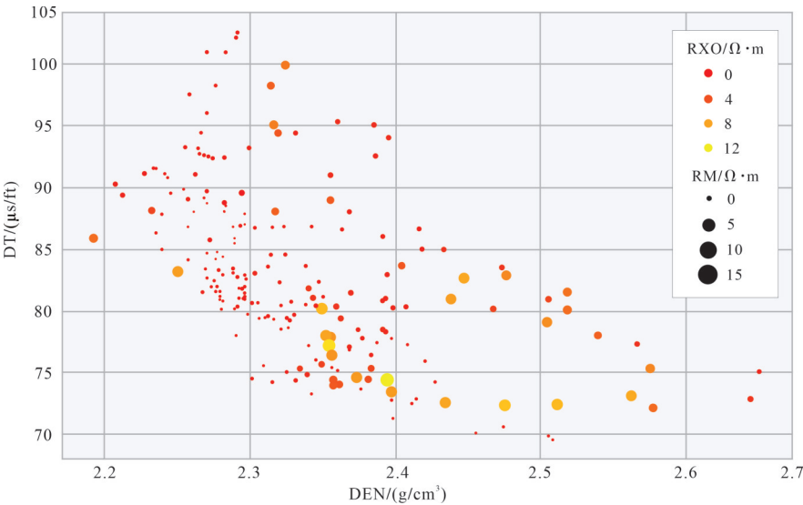
图8 沥青测井参数气泡图
