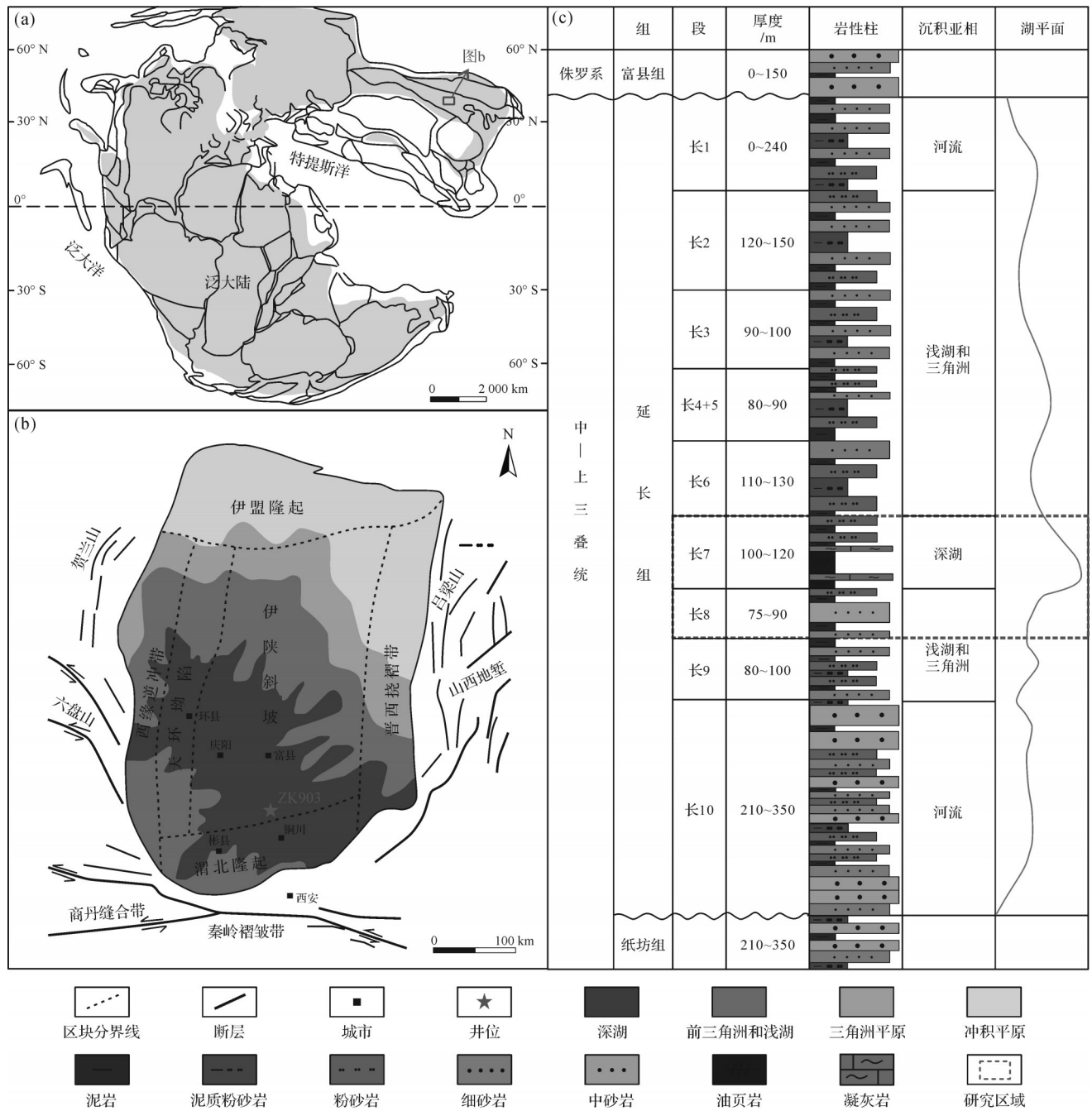
图1 鄂尔多斯盆地区域地质图
