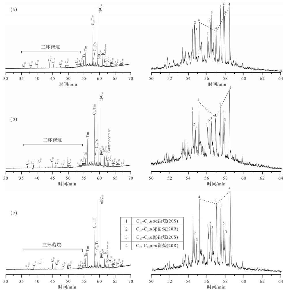
图3 鄂尔多斯盆地长7段—长8段饱和烃( m/z 191及217)萜烷与甾烷质量色谱图 (a)ZK903井,长8段,806.95 m,TOC:5.81%;(b)ZK903井,长7 3 段,754.50 m,TOC:9.06%;(c)ZK903井,长7 1+2 段,689.81 m,TOC:10.45%;
