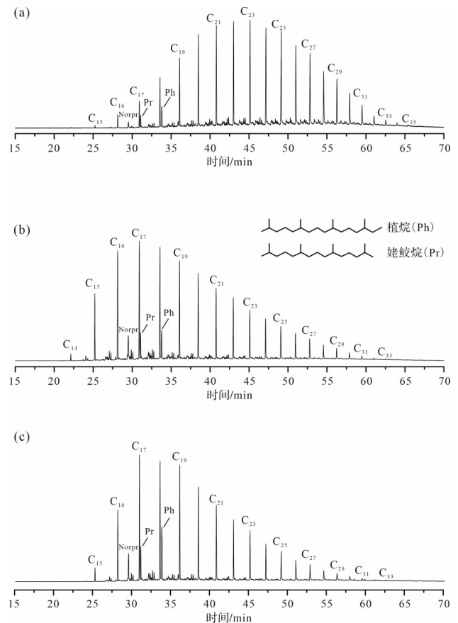
图2 鄂尔多斯盆地长7段—长8段饱和烃( m/z 57)正构烷烃质量色谱图
