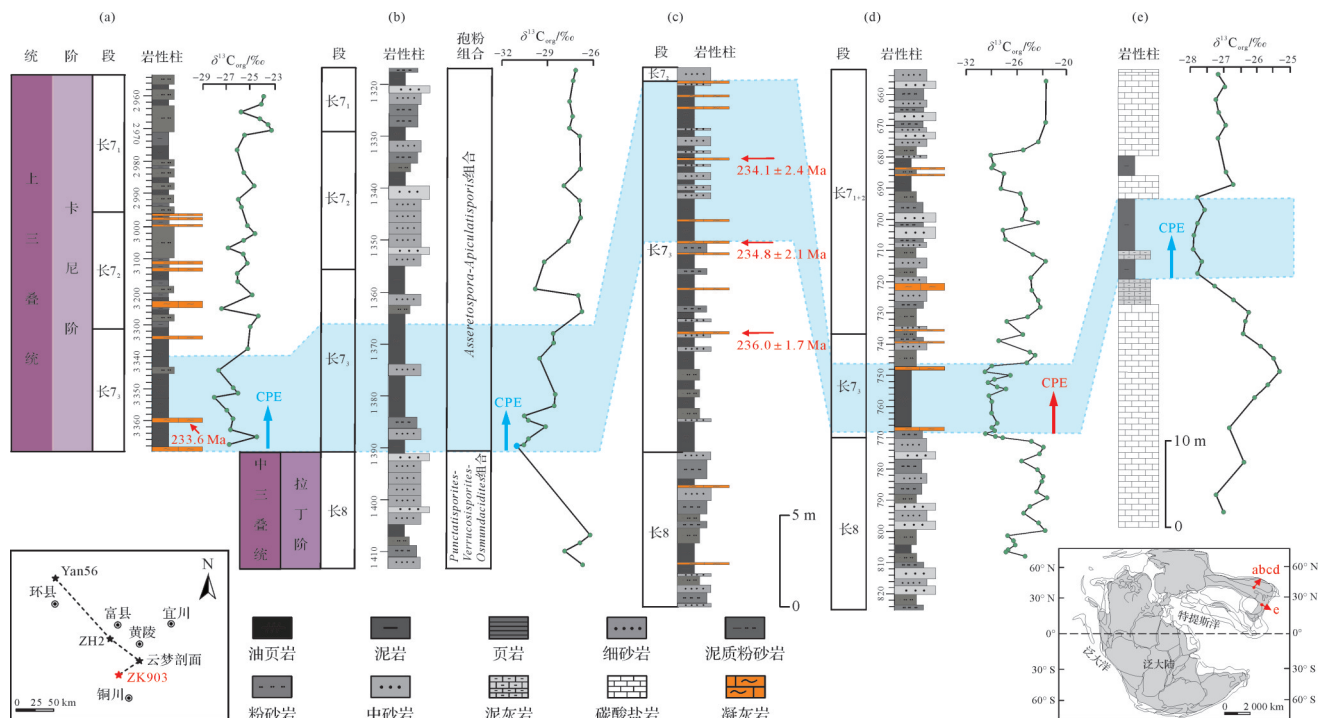
图 4 卡尼期地层对比
