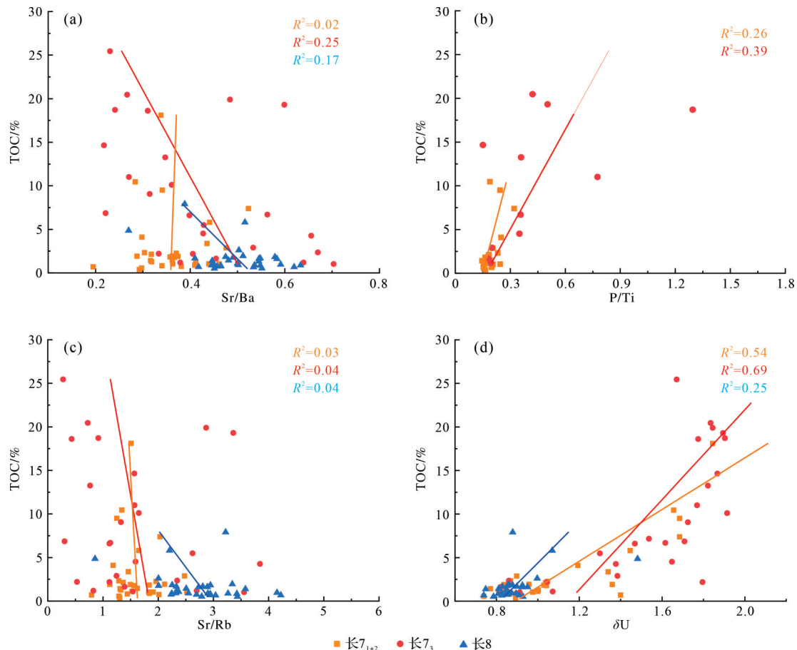
图 9 鄂尔多斯盆地长 7 段—长 8 段样品 TOC 与各环境指标的相关性图
