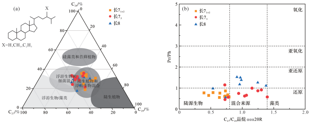
图8 鄂尔多斯盆地长7段—长8段有机质来源判别图
