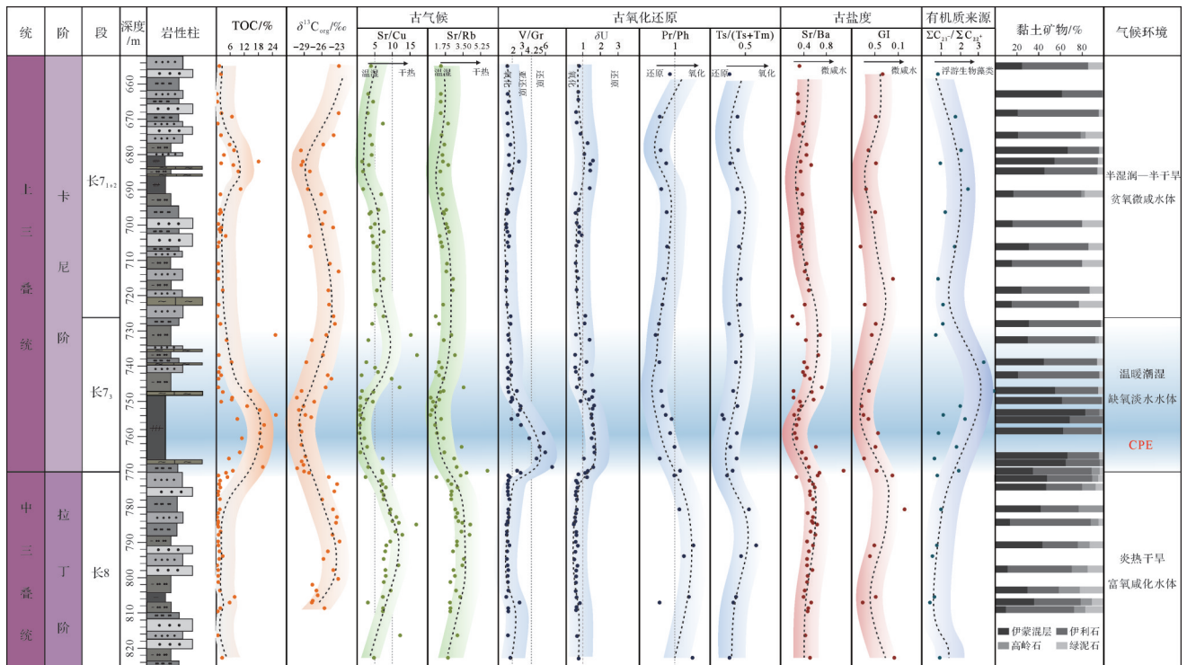
图5 鄂尔多斯盆地长7段—长8段古气候与沉积环境综合柱状图
