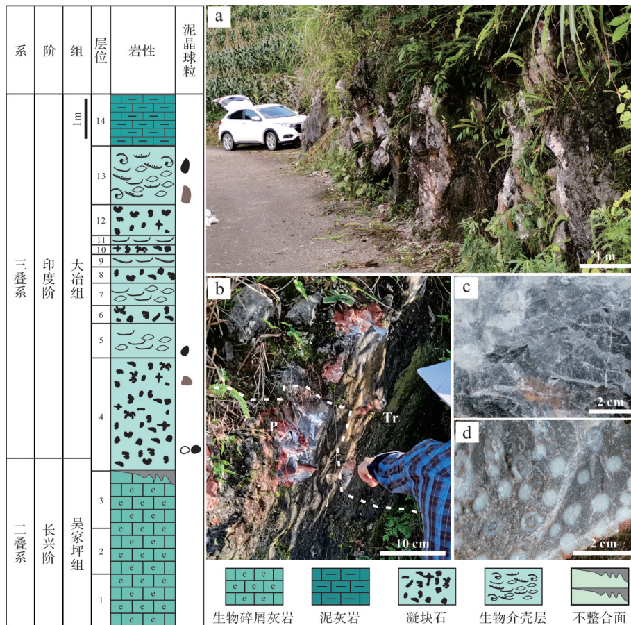
图2 田湾剖面微生物岩序列的岩性柱状图以及典型岩性类型的野外露头
