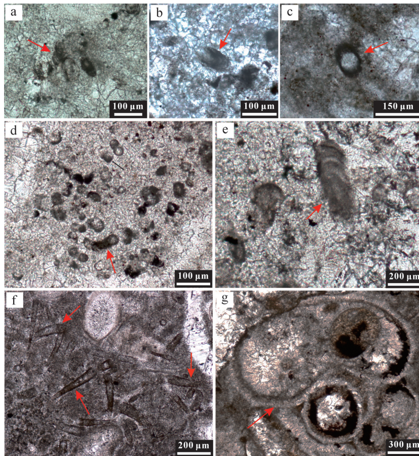
图4 田湾剖面微生物岩中微生物和后生生物化石的显微特征
