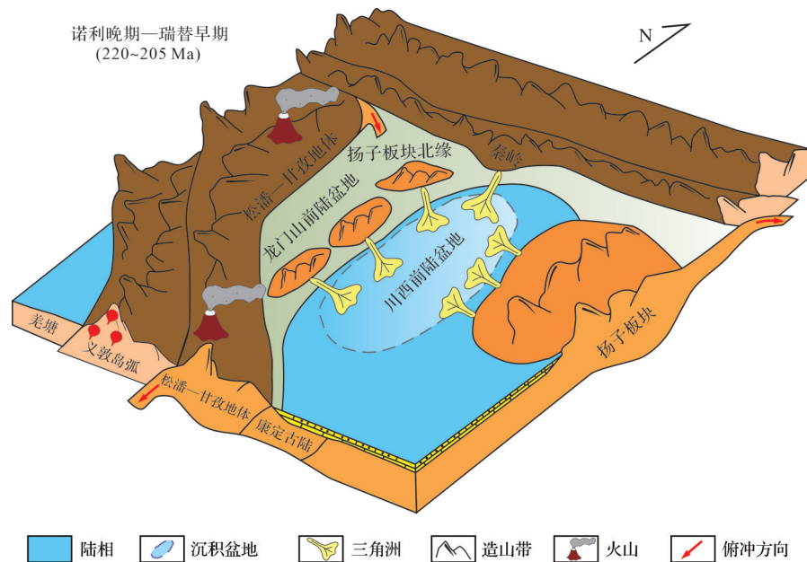
图 12 扬子板块西缘晚三叠世构造演化模式图 (据 Gou et al. , 2024 修改)
