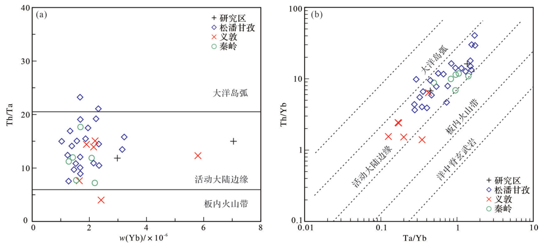
图 11 构造环境判定图 (据 Gorton and Schandl, 2000 修改)
