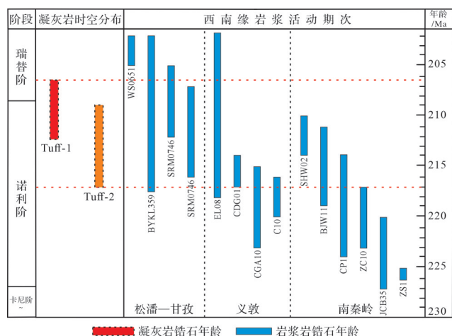
图7 须家河组凝灰岩时空分布图
