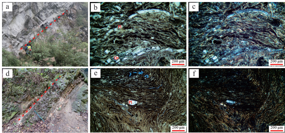
图3 鸡冠山剖面凝灰岩特征
