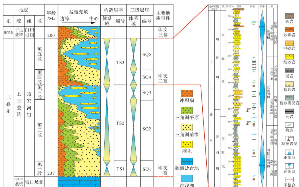
图2 鸡冠山剖面须家河组综合柱状图(据郑荣才等, 2009; 陈杨, 2011 修改)
