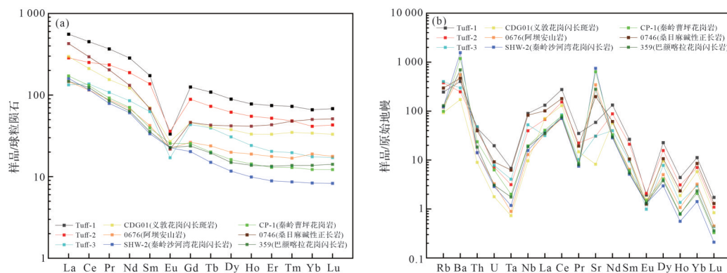
图6 (a)球粒陨石标准化稀土配分曲线图;(b)原始地幔标准化微量元素蛛网图
