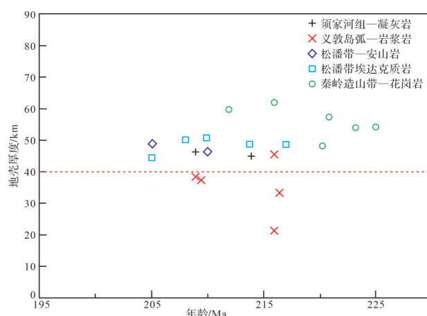
图10 地壳厚度与锆石年龄关系图 义敦岛弧岩浆岩数据引自文献(施滔, 2017), 松潘安山岩和埃达克质岩数据引自文献(蔡宏明, 2010; 李成祥等, 2023; 王鹏等, 2023), 秦岭花岗岩数据引自文献(弓虎军等, 2009; 刘巍等, 2020)
