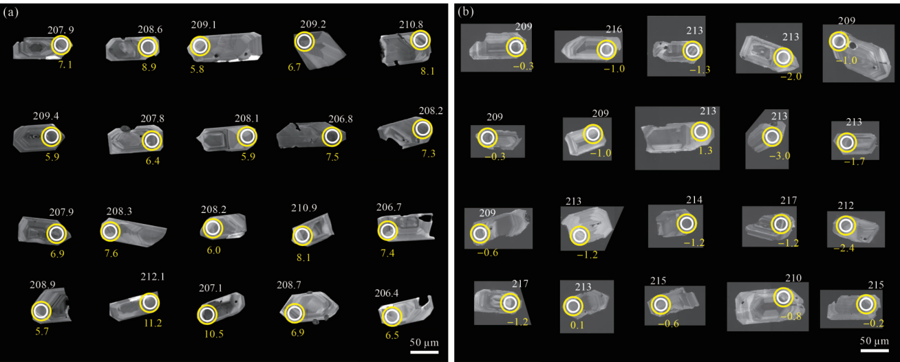
图4 样品锆石阴极发光图像
