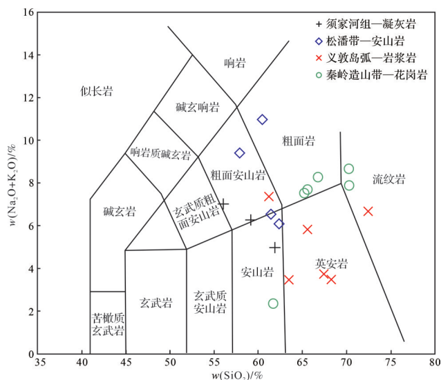
图8 须家河组凝灰岩母岩判别图 (据 Le Bas et al. , 1986 修改)
