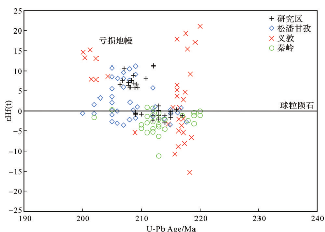
图9 须家河组凝灰岩锆石 U-Pb 年龄和 \epsilon_{\text{Hf}}(t) 图解 松潘岩体数据引自文献(蔡宏明, 2010; 王鹏等, 2023), 义敦岛弧岩体数据引自文献(施滔, 2017), 秦岭岩体数据引自文献(弓虎军等, 2009; 刘巍等, 2020)
