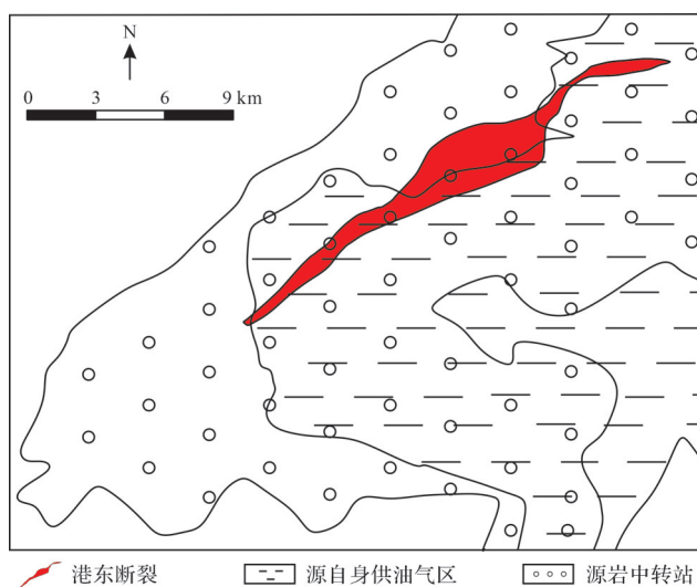
图4 港东断裂与沙三段源岩中转站和自身供油气区分布关系图
