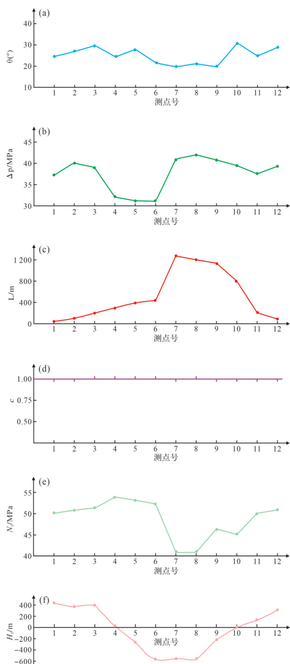
图3 明化镇组沉积中晚期穿过沙一中亚段港东断裂向东三段输导油气能力指数计算参数分布特征图
