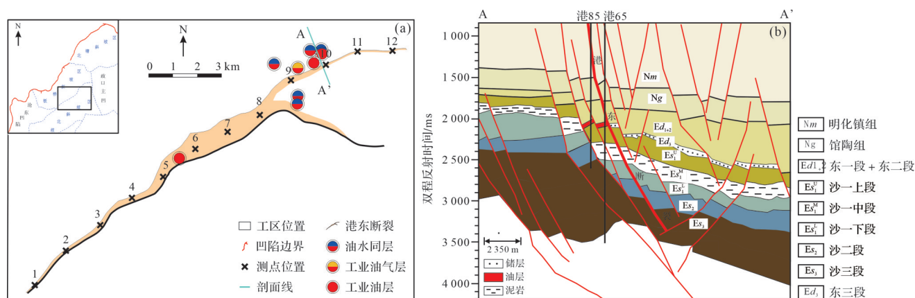
图2 港东断裂处东三段油气分布关系图
