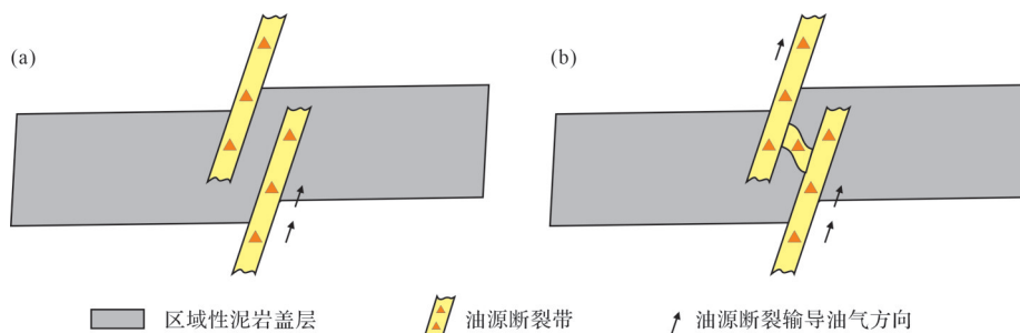
图1 泥岩盖层减弱油源断裂输导油气能力程度示意图
