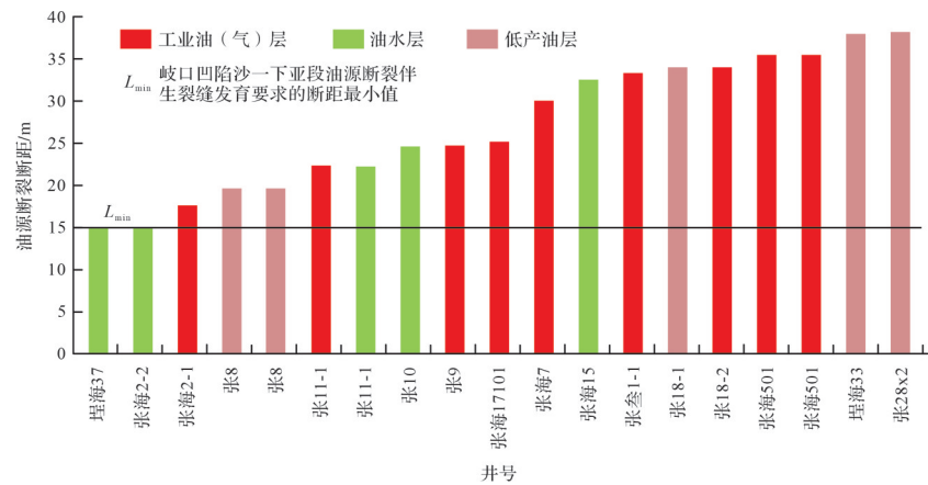
图5 歧口凹陷沙一下亚段内油源断裂伴生裂缝发育要求的断距最小阈值厘定图
