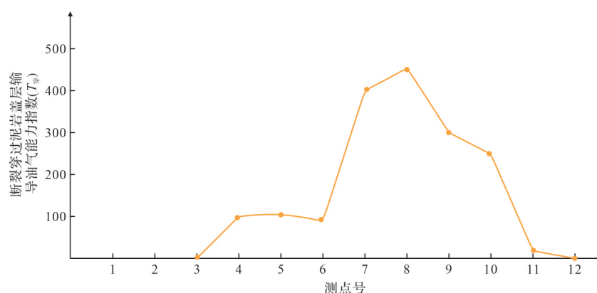
图8 港东断裂穿过沙一中亚段区域性泥岩盖层输导油气能力指数分布图
