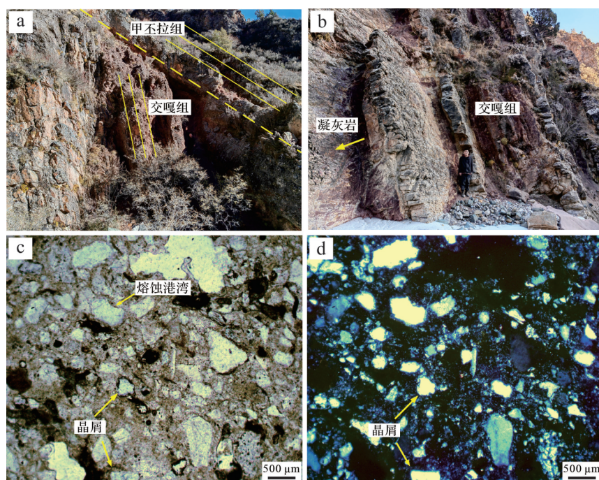
图4 王卡剖面凝灰岩特征
