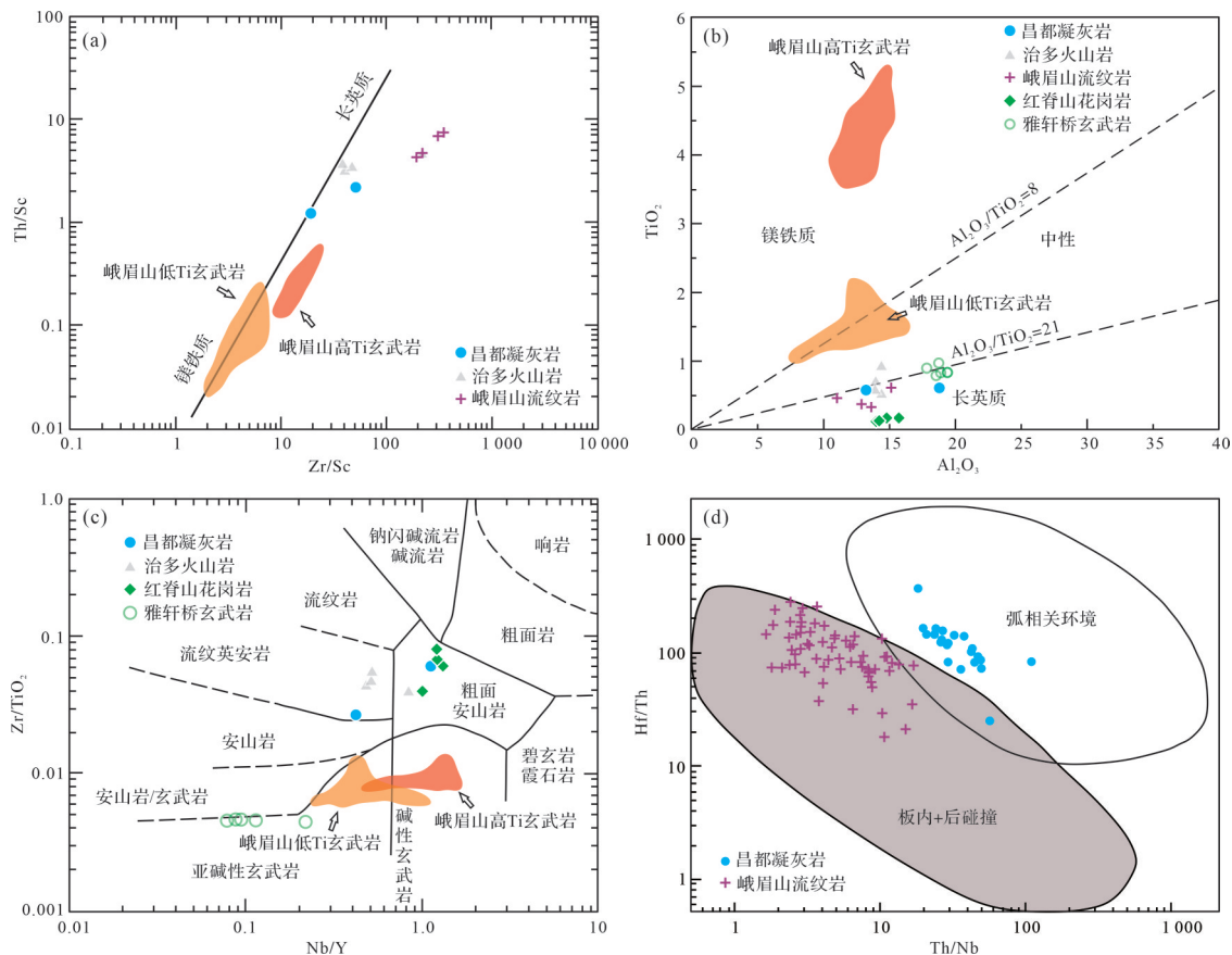
图8 (a)全岩 Zr/Sc-Th/Sc 图解; (b)全岩 \text{Al}_2\text{O}_3 - \text{TiO}_2 图解; (c)全岩 Nb/Y-Zr/ \text{TiO}_2 图解; (d)锆石 Th/Nb-Hf/Th 图解 红脊山花岗岩全岩微量元素数据引自张乐等(2014), 治多区域岩浆岩全岩微量元素数据引自 Yang et al. (2011), 雅轩桥玄武岩全岩微量元素数据引自 Fan et al. (2010), 峨眉山高Ti和低Ti全岩微量元素数据引自 Huang et al. (2022a), 峨眉山流纹岩锆石微量和全岩微量数据引自 Huang et al. (2022a)
