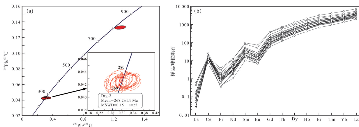
图6 (a) 锆石 U-Pb 年龄谐和曲线; (b) 锆石球粒陨石标准化稀土元素配分模式
