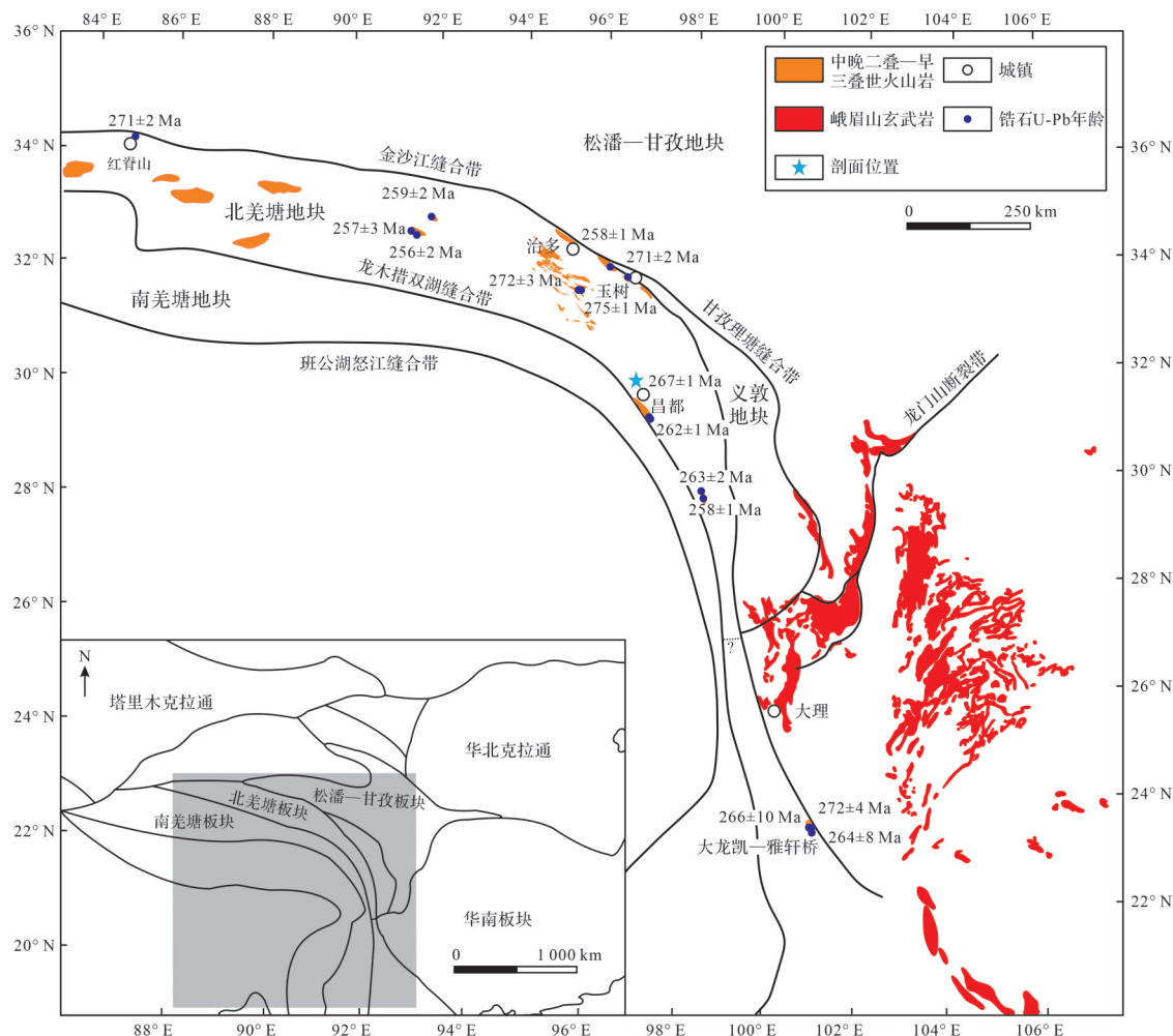
图 1 研究区地质构造简图(据沈树忠等, 2024 修改)
