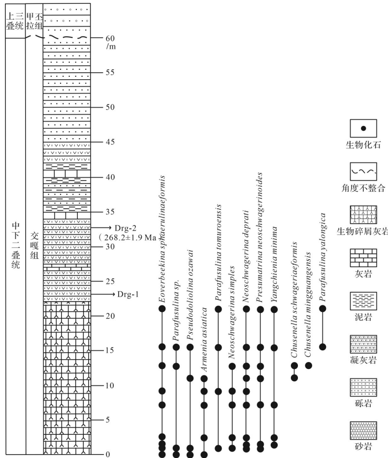
图3 北羌塘地块昌都地区王卡剖面地层柱状图(据 Qiao et al. , 2021 修改)
