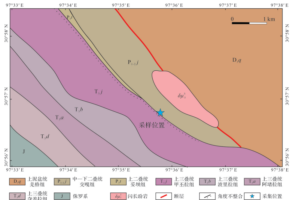
图2 北羌塘地块昌都地区王卡剖面地质简图(据陈丰琪和钟康惠,2013修改)
