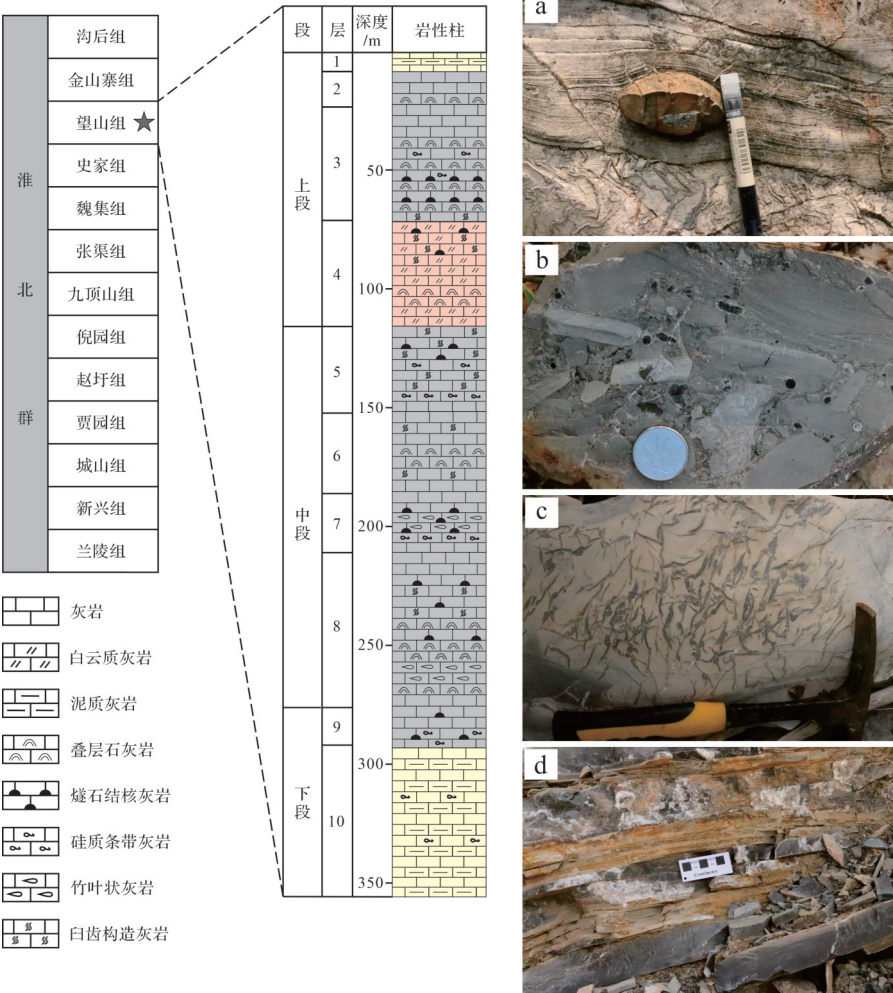
图 2 望山组实测地层柱状图及露头剖面
