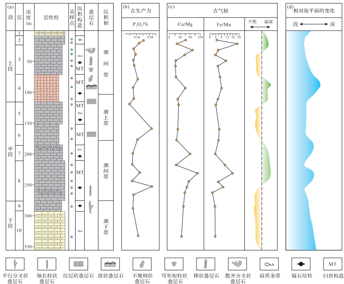
图8 徐淮地区望山组古环境演化图
