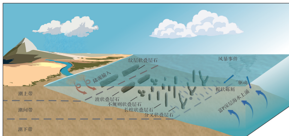
图9 徐淮地区望山组沉积模式图
