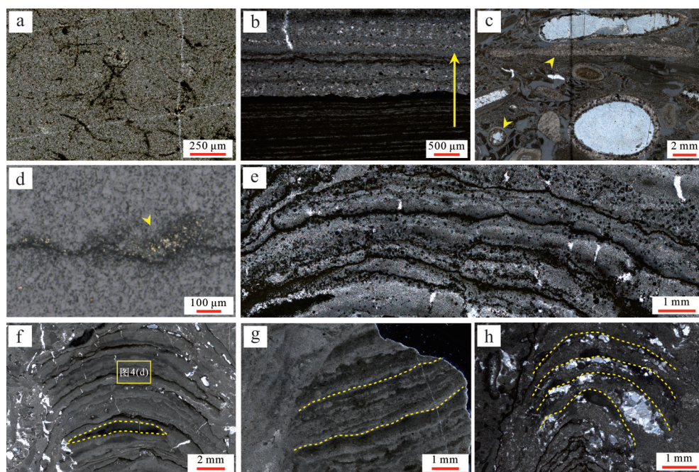
图4 徐淮地区望山组叠层石显微镜下特征
