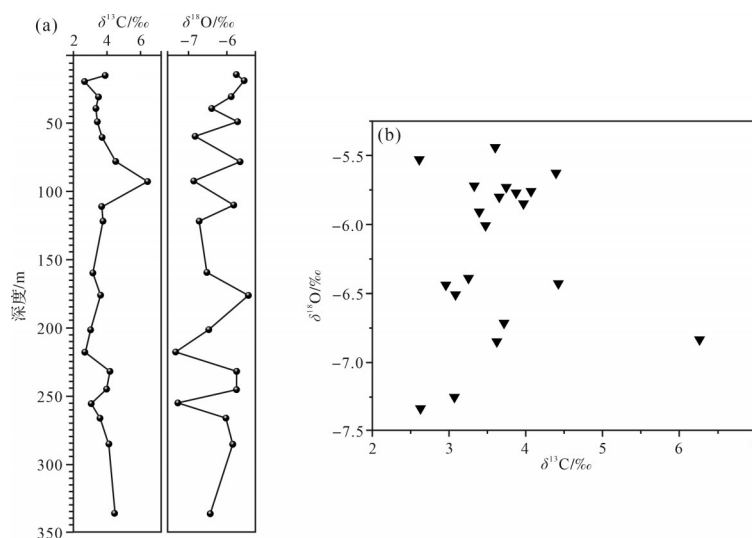
图7 徐淮地区望山组样品 \delta^{13}\text{C} 、 \delta^{18}\text{O} 及其相关性
