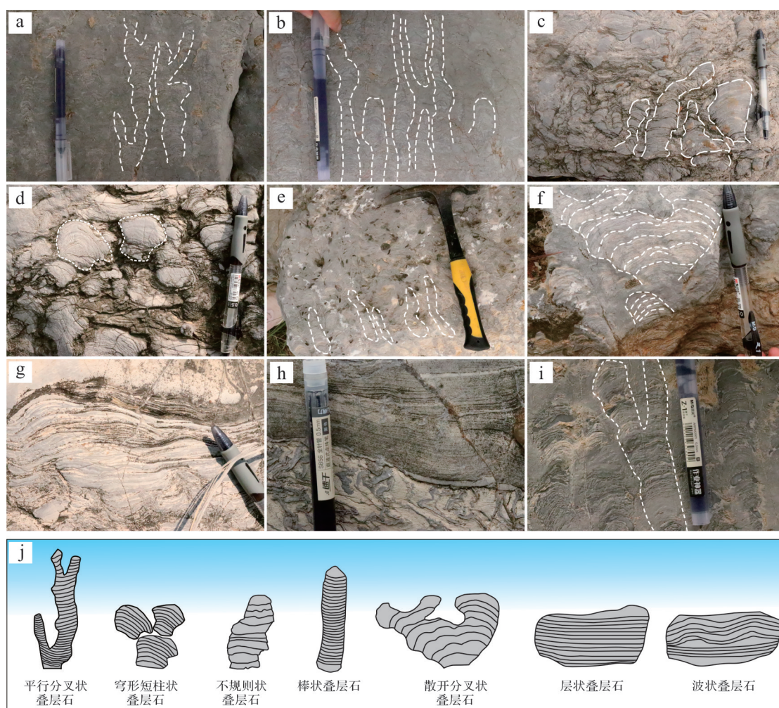
图3 徐淮地区望山组叠层石类型及宏观特征
