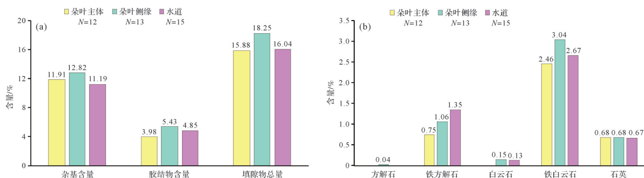
图6 庆城地区长 7_{1-2} 亚段砂岩填隙物(a)及胶结物类型(b)分布柱状图
