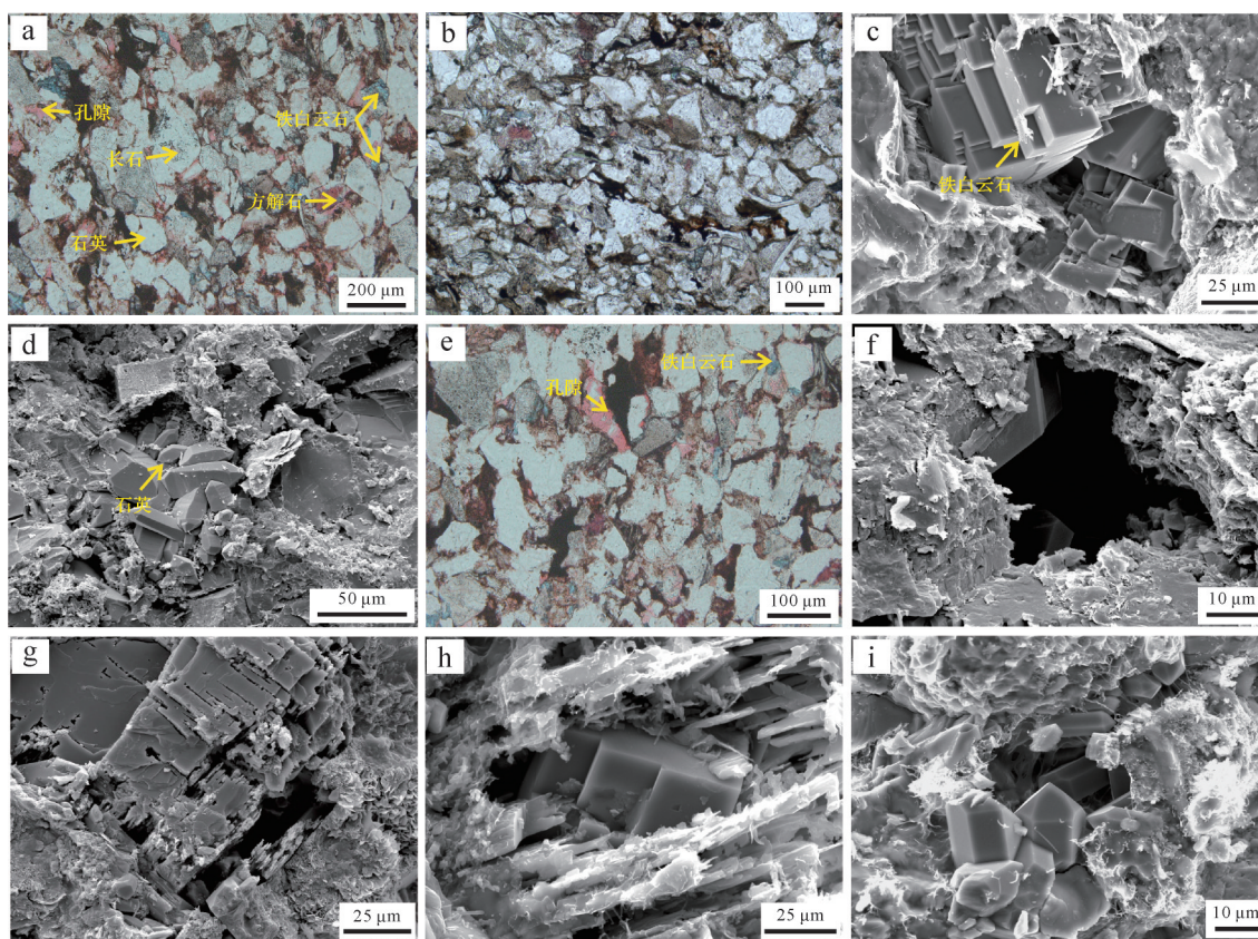
图7 庆城地区长 7_{1-2} 亚段砂岩岩石学特征图
