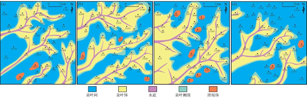
图3 鄂尔多斯盆地Z185区长7 1-2 亚段沉积微相图 (a)长7 1 小层沉积微相图;(b)长7 2 小层沉积微相图;(c)长7 2 小层沉积微相图;(d)长7 2 小层沉积微相图 Fig. 3 Sedimentary microfacies diagram of Chang 7 1-2 sub-member in Z185 area, Ordos Basin
