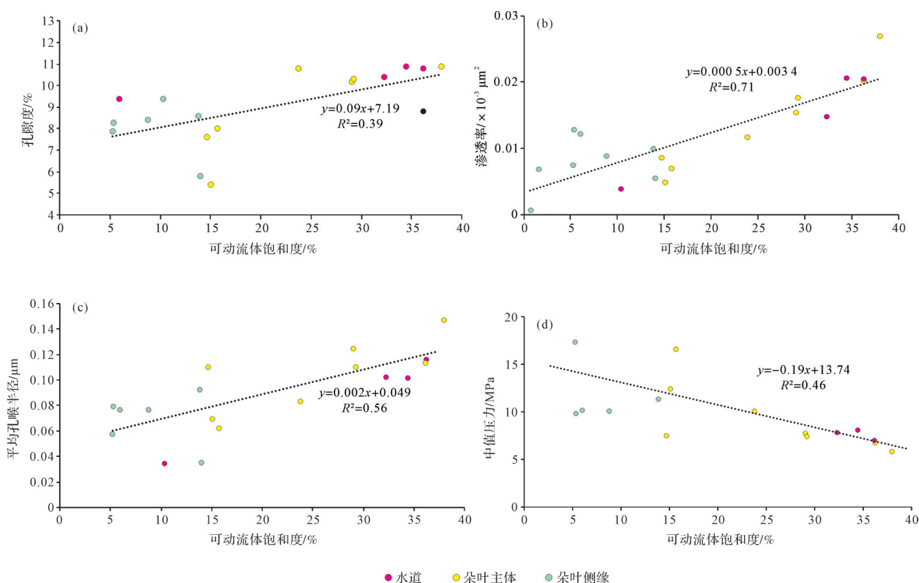
图13 庆城地区长7 1-2 亚段砂岩可动流体饱和度与物性(a,b)和孔隙结构参数关系(c,d)散点图
