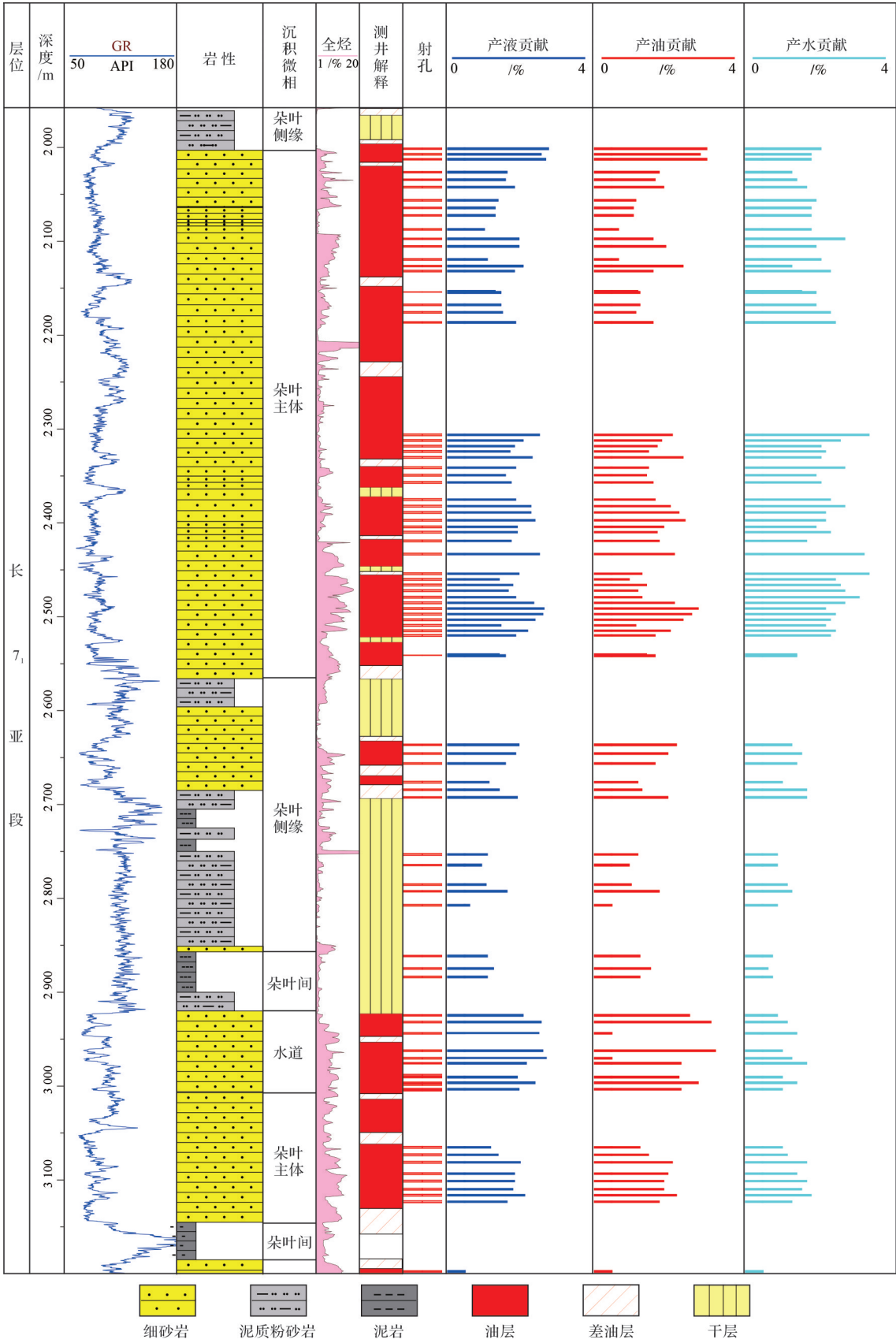
图 16 Q41-4 水平段综合柱状图 Fig. 16 Comprehensive histogram of Q41-4 horizontal section
