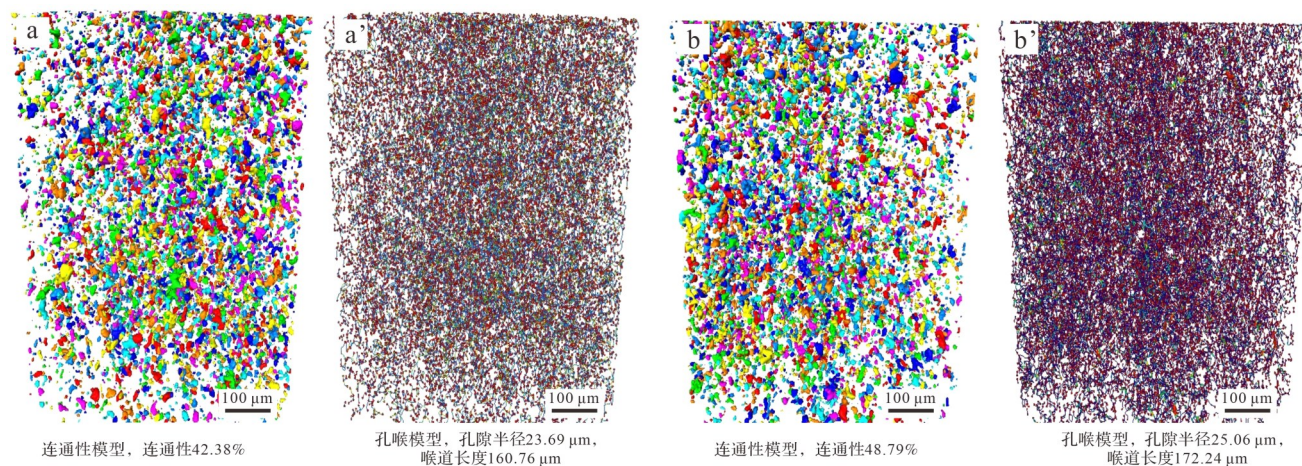
图9 庆城地区长 7_{1-2} 亚段砂岩微米CT扫描模型
