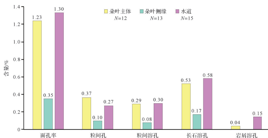
图8 庆城地区长 7_{1-2} 亚段砂岩孔隙类型分布柱状图
