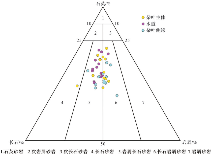
图5 庆城地区长7 1,2 亚段砂岩类型三角图 Fig. 5 Sandstone type triangle diagram of Chang 7 1,2 sub-member, Qingcheng area
