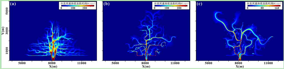
图 5 模拟三角洲分流河道网络分布特征
