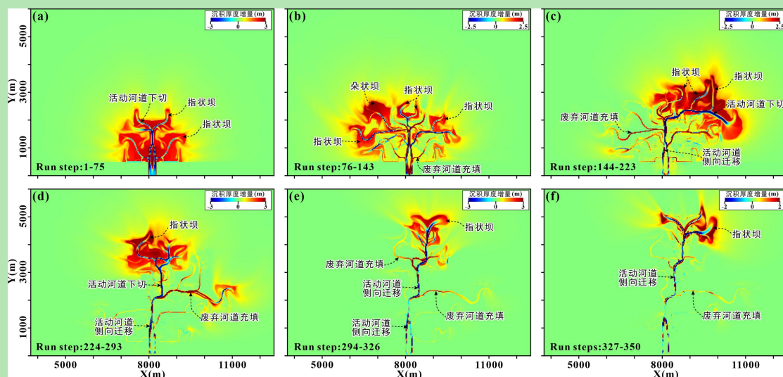
图 9 砂泥质浅水三角洲增生演化过程 (Run 2)
