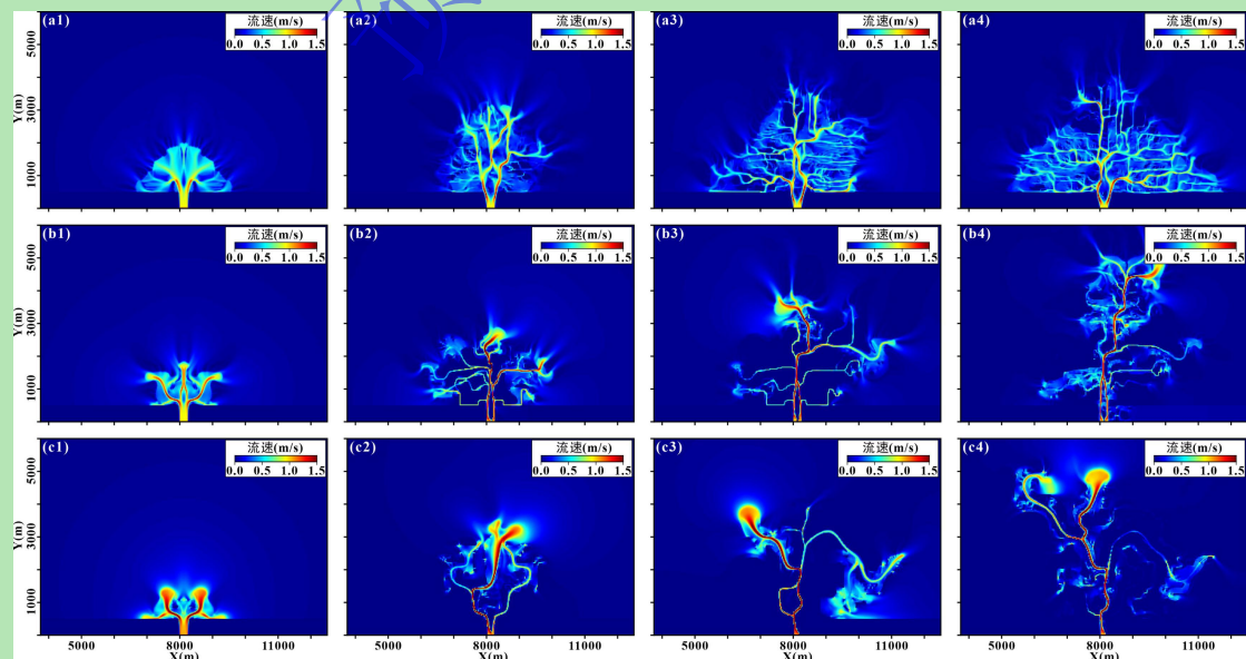
图 4 模拟三角洲流速分布特征
