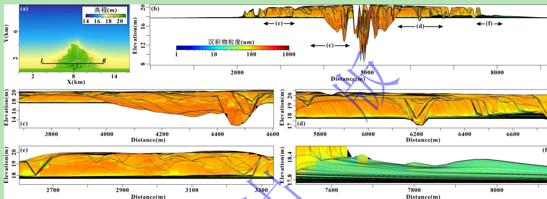
图 8 富砂质浅水三角洲物源方向沉积构型特征与沉积物粒度分布 (Run 1)
