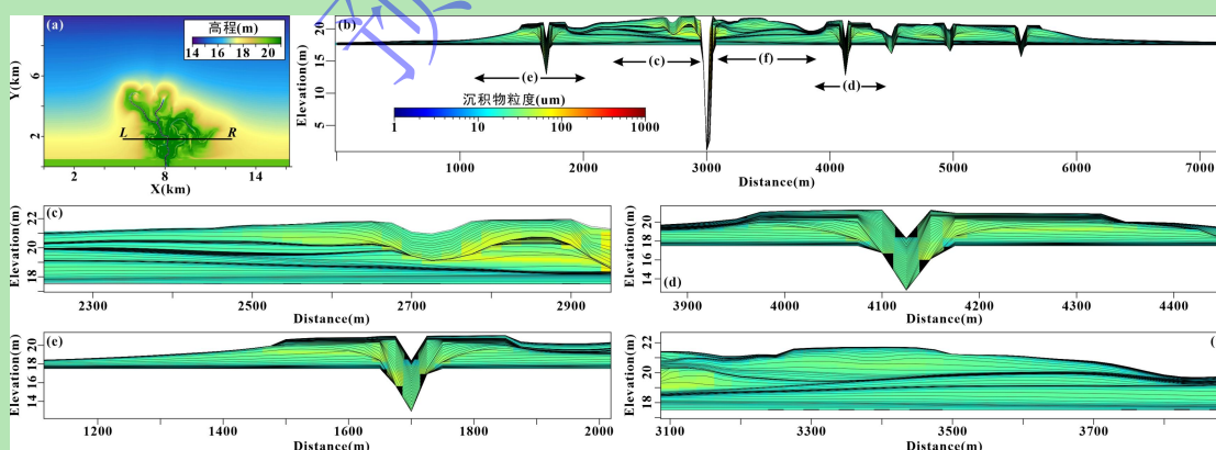
图 12 富泥质浅水三角洲沉积构型特征与沉积物粒度分布 (Run 3)
