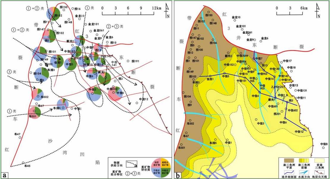
图5 中拐凸起佳木河组沉积期重矿物与沉积相展布图
