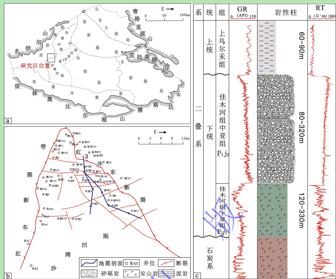
图 1 中拐凸起构造背景及佳木河组纵向岩性发育特征
