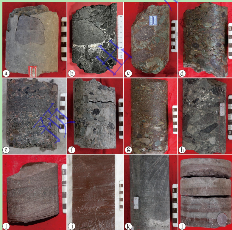
图 3 中拐凸起及周缘主要岩相类型
