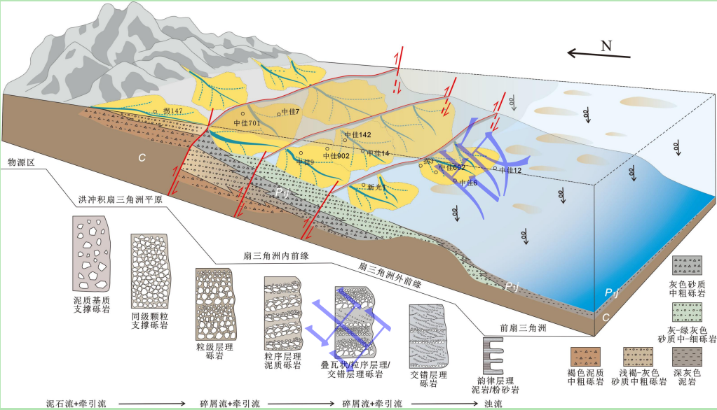
图 7 中拐凸起佳木河组断阶型扇三角洲沉积模式
