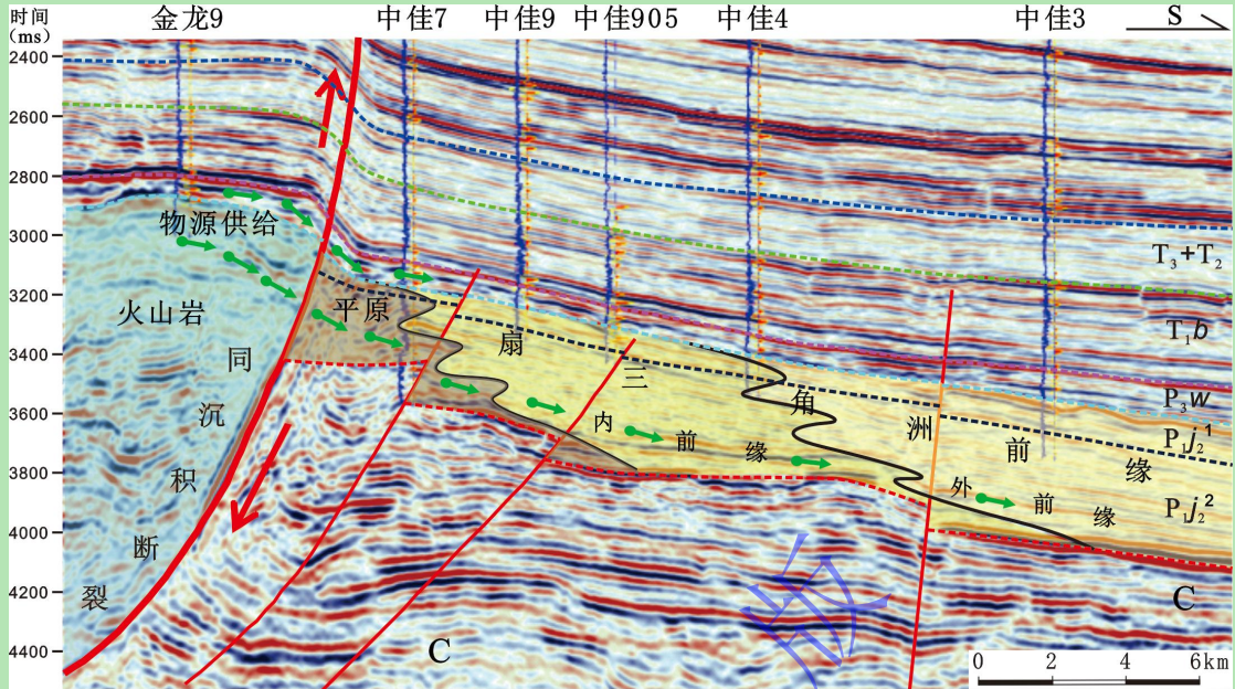
图8 垂直红3井东断裂带佳木河组最大主物源方向地震剖面
