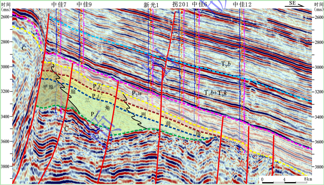
图9 中拐凸起凹陷区断阶分布地震示意图
