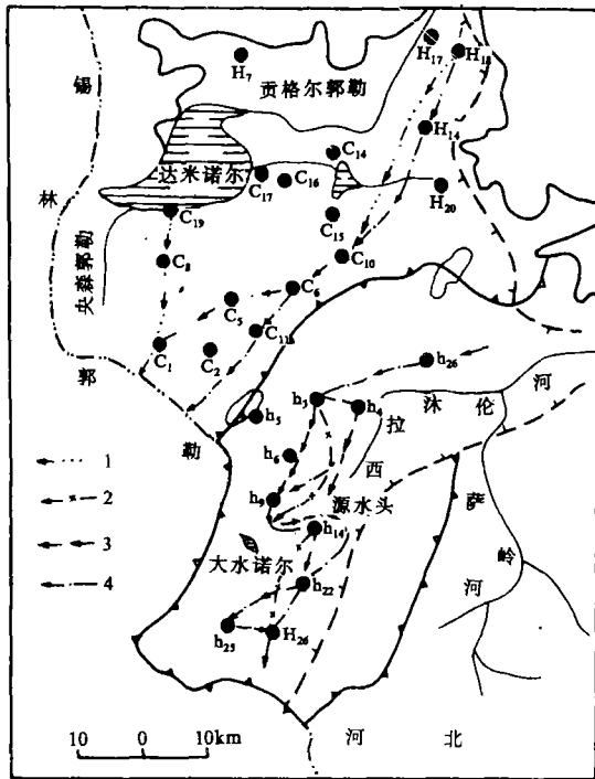
1、中更新世主要河道 2、中更新世初期主要河道 3、中更新世晚期主要河道 4、晚更新世初期主要河道
