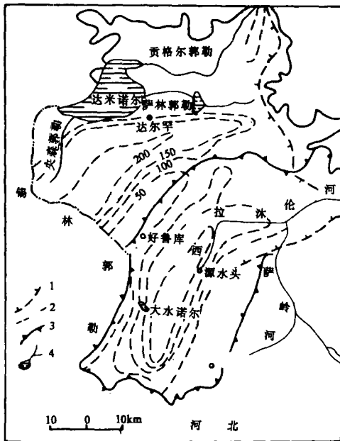
1.盆地界线 2.等厚线 3.地表分水岭 4.河湖
