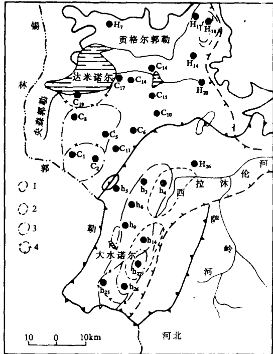
1、中更新世中期湖区 2、中更新世末期湖心区 3、晚更新世中期湖心区 4、晚更新世末期湖心区
