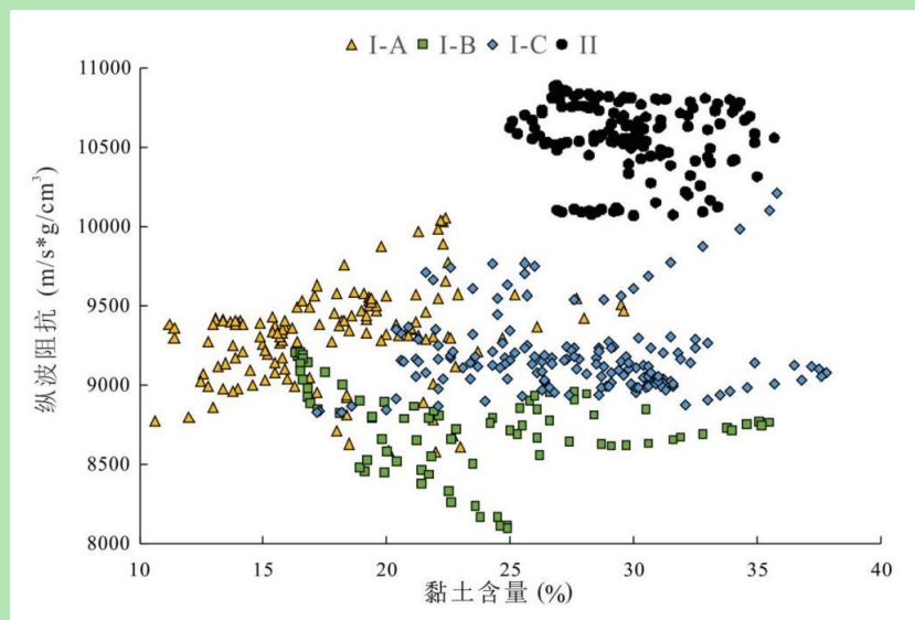
图 4 W01 井龙马溪组页岩纵波阻抗与黏土含量交会图（数据按沉积单元排列）
