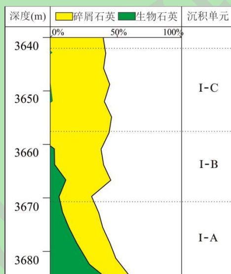
图 7 W01 井龙马溪组页岩石英成分和含量垂直变化图
