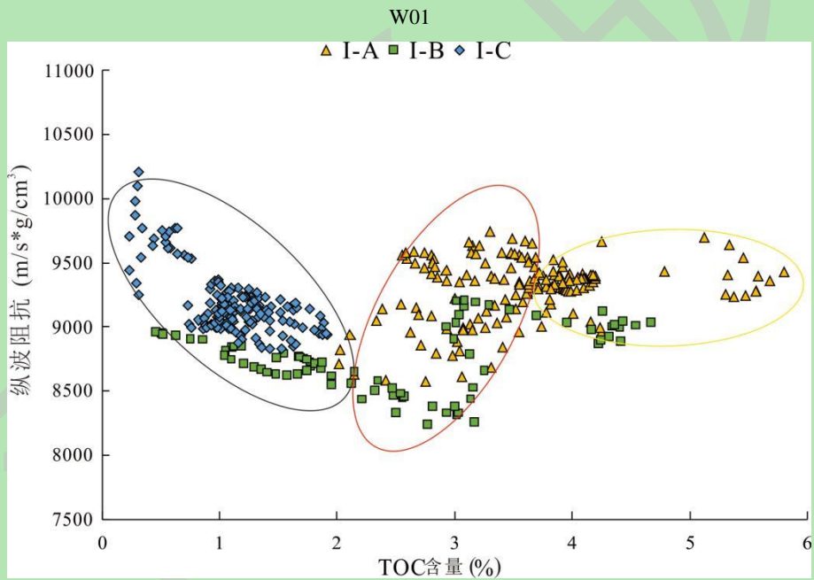
图9 W01井龙马溪组页岩 TOC 含量与纵波阻抗交会图
