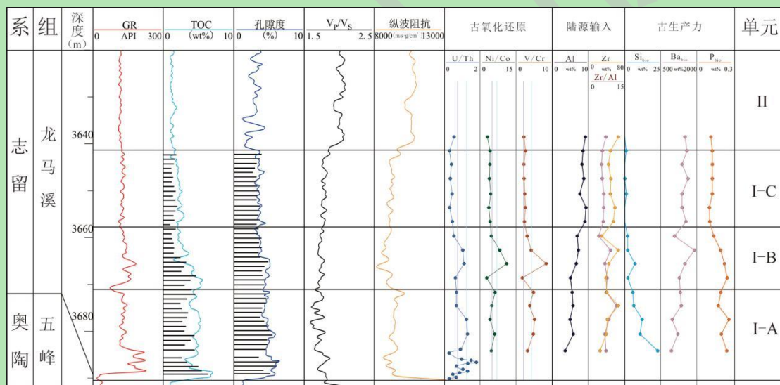
图2 W01井龙马溪页岩沉积单元综合柱状图
