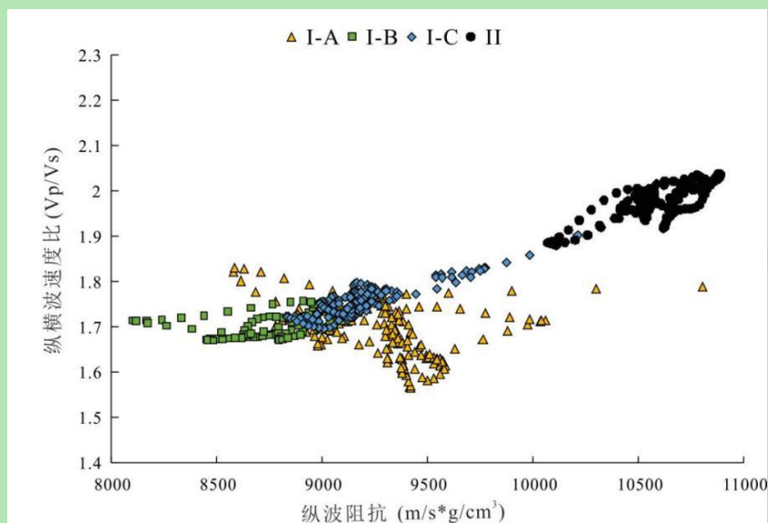
图6 W01井龙马溪组页岩纵波阻抗与纵横波速度比交会图(数据按沉积单元排列)
