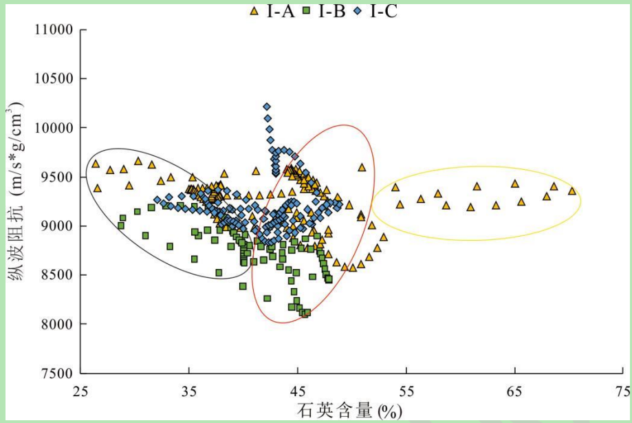
图8 W01井龙马溪组页岩石英含量与纵波阻抗交会图
