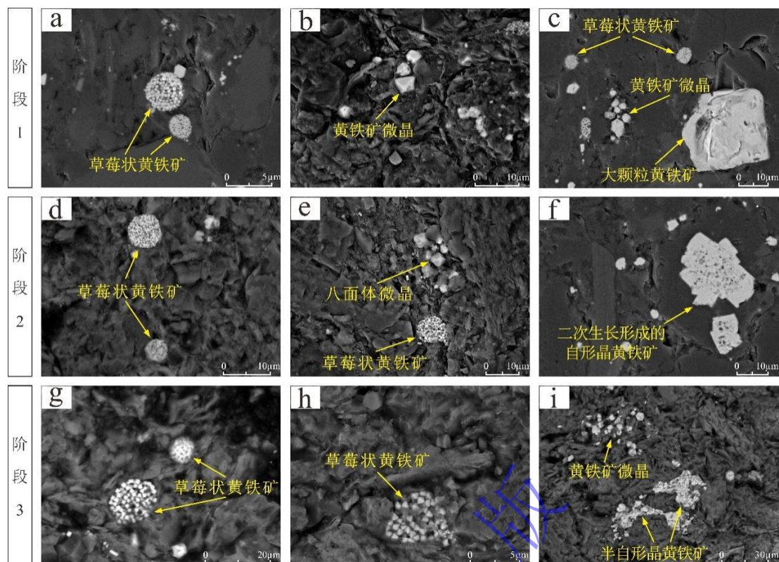
图3 W207井筇竹寺组扫描电镜下黄铁矿形态
