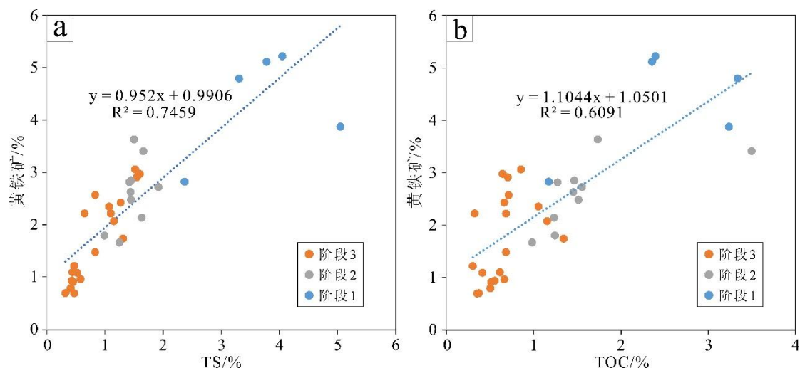
图2 W207井筇竹寺组黄铁矿与TS、TOC含量相关性分析
