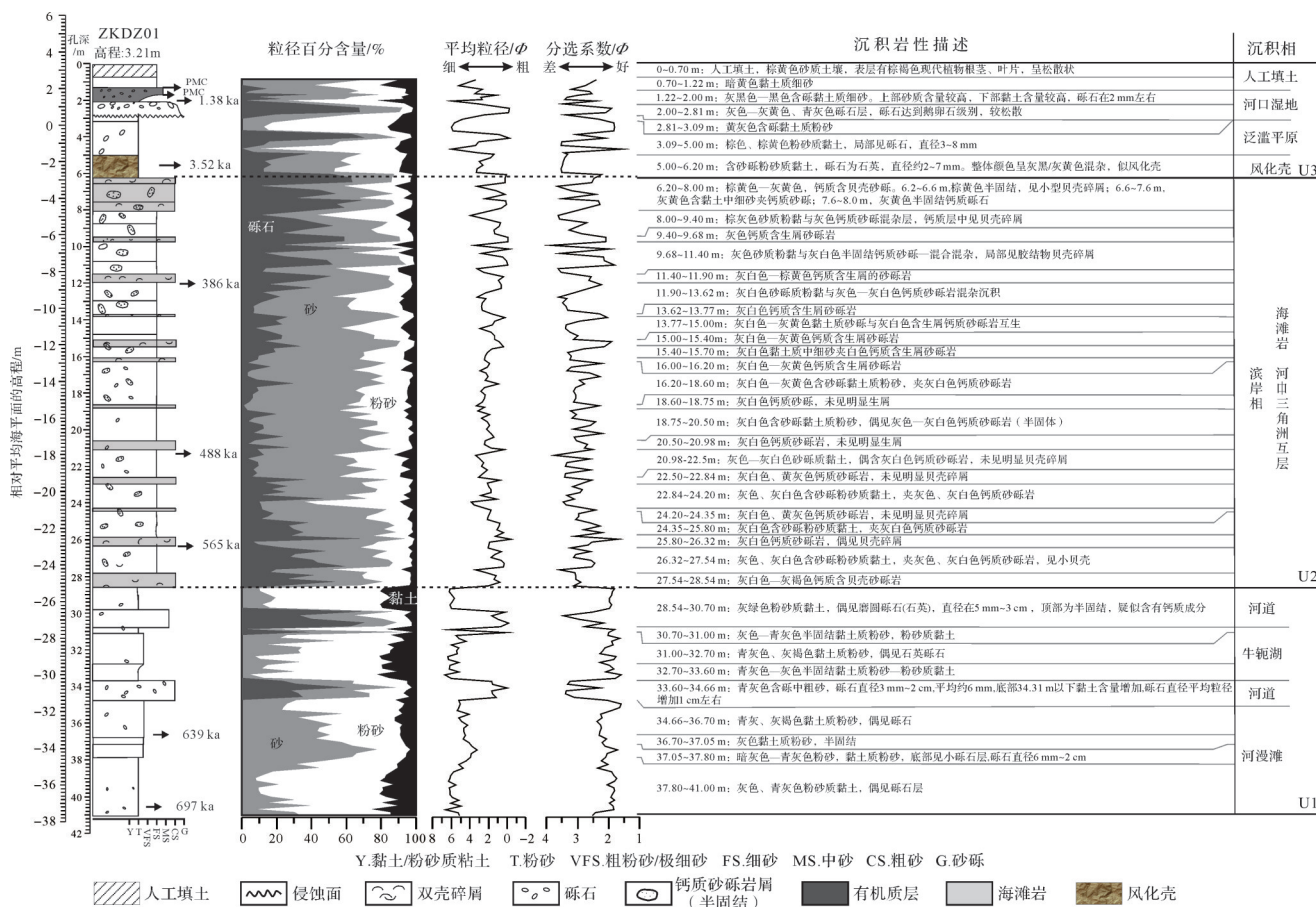
图2 ZKDZ01 钻孔综合柱状图(Zhu et al. , 2026)
