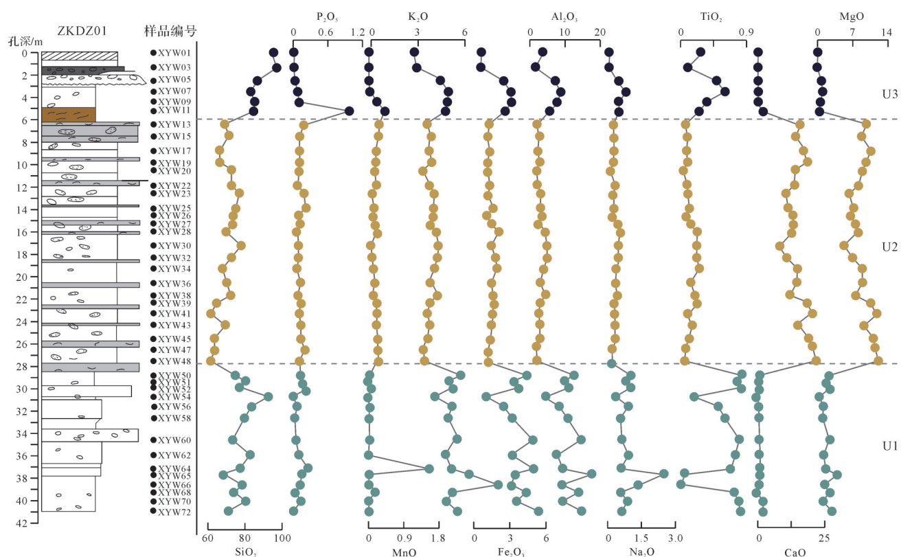
图3 ZKDZ01 钻孔主量元素含量变化图
