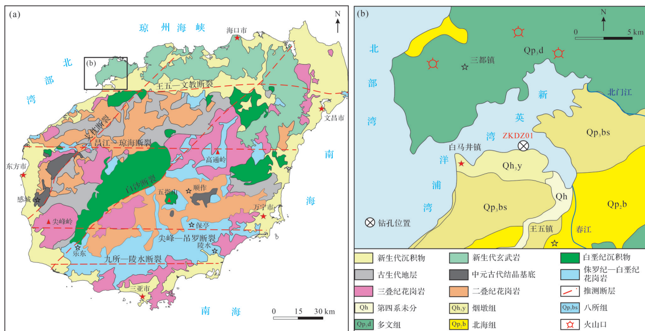
图1 (a)海南岛区域地质图(张磊等,2022);(b)新英湾ZKDZ01钻孔位置图(Zhu et al. , 2026)
