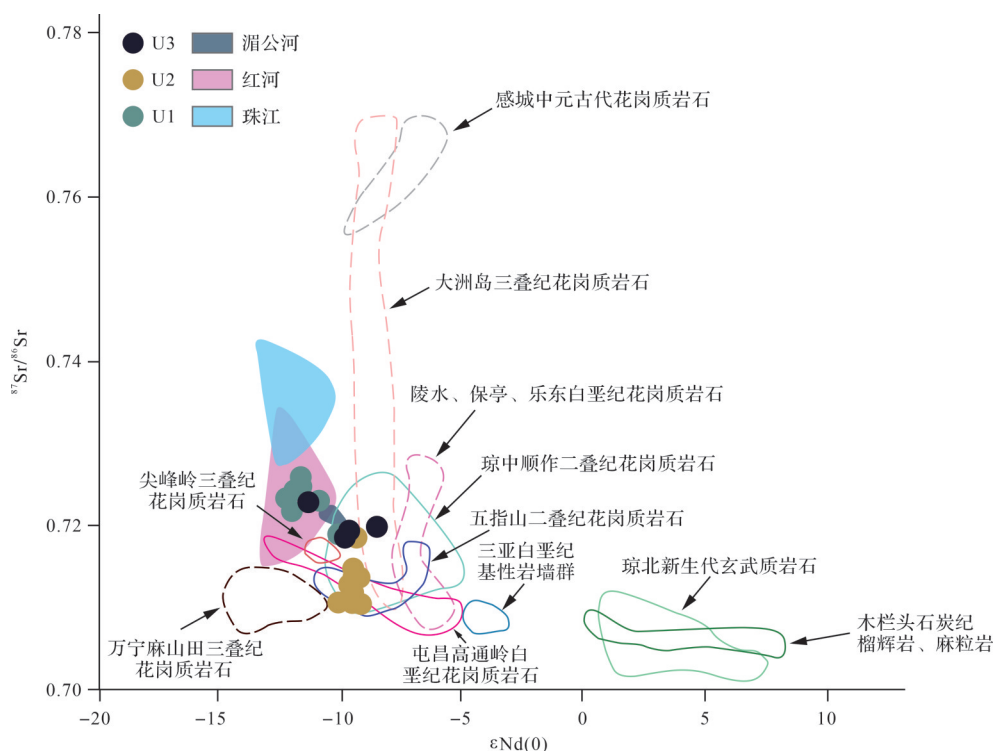
图7 ZKDZ01 钻孔沉积物 ^{87}\text{Sr}/^{86}\text{Sr} - \epsilon_{\text{Nd}(0)} 判别图解 (Liu et al. , 2007; 张磊等, 2022)
